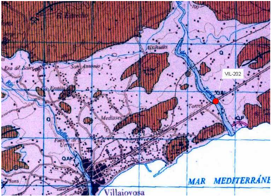
Mapa geológico
