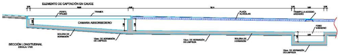
Avenida de Finestrat antes de la confluencia con Avda. Marina Baixa. Cámara de laminación
