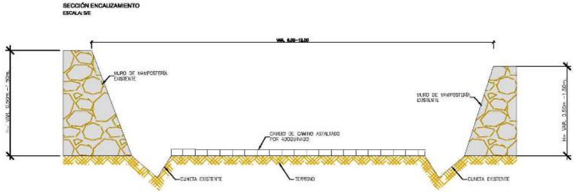
Avenida de Finestrat. Sección tipo canal abierto
