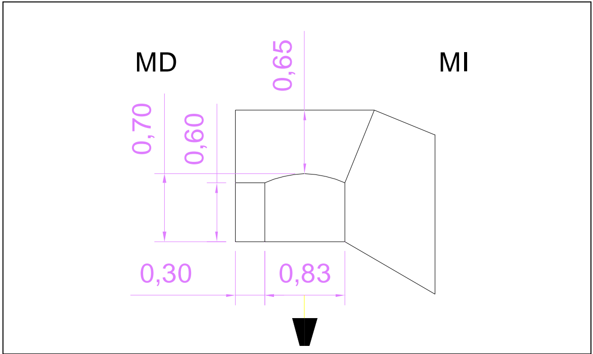
Situación actual de la obra de paso BEN-107
