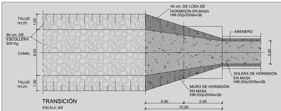
Detalle de los areneros para retención de sólidos
