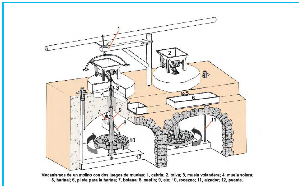
Esquema de un molino de dos muelas
