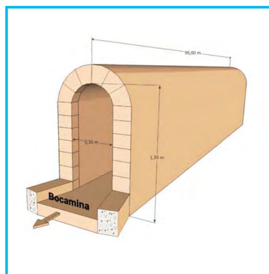
Esquema de un minado de transporte
