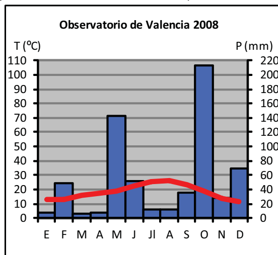
Diagrama climático del Observatorio termopluviométrico de València
