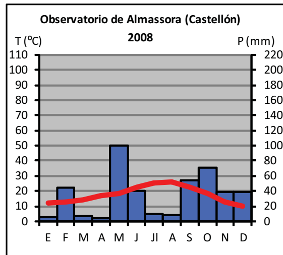
Diagrama climático del Observatorio termopluviométrico de Almassora
