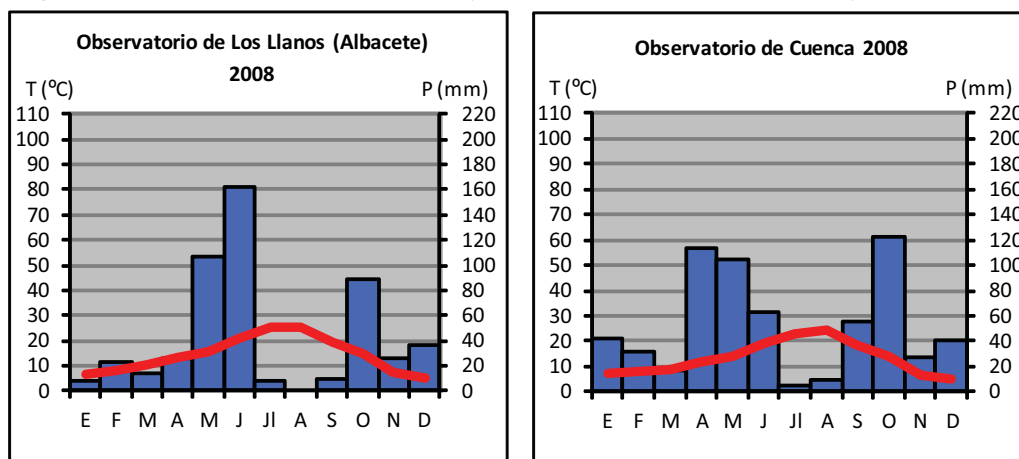
Diagramas climáticos de los Observatorios termopluviométricos de Los Llanos (Albacete) y de Cuenca
