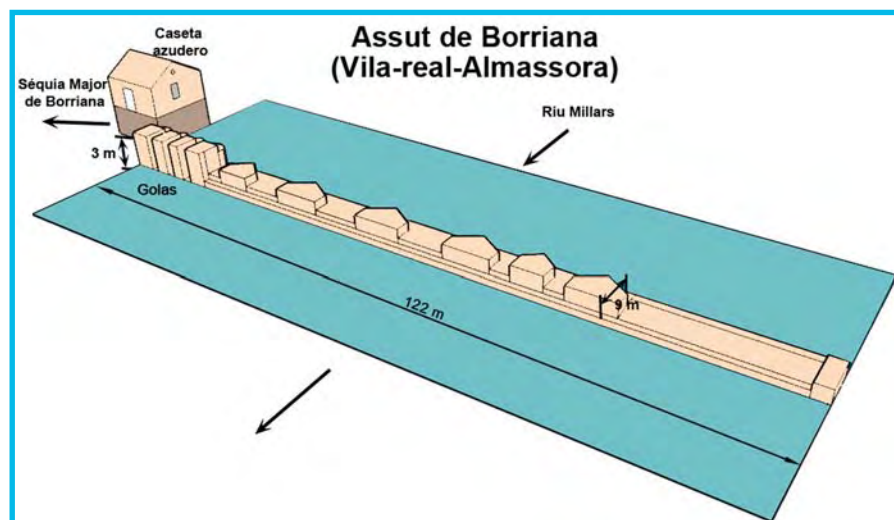
Esquema de un Azud
