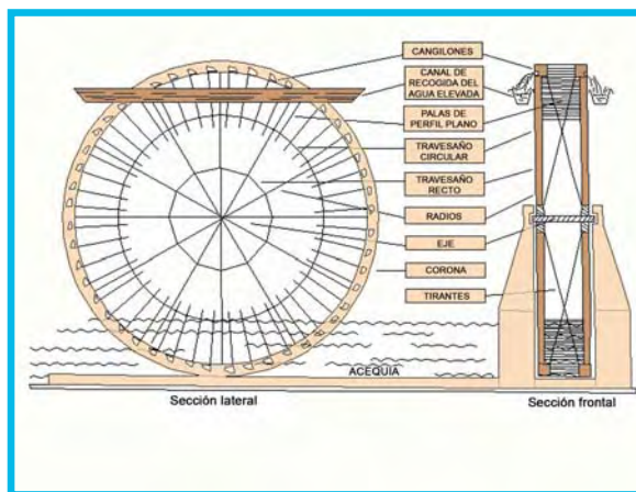
Esquema de una Noria Fluvial
