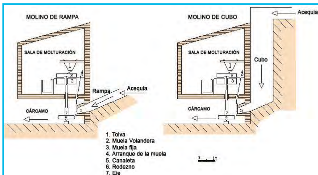
Esquema de funcionamiento de un molino harinero
