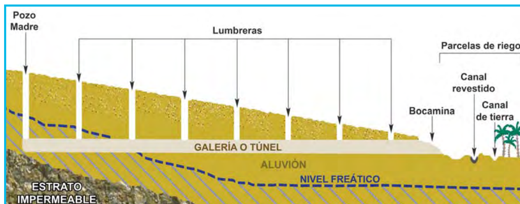
Esquema de funcionamiento de un Qanat
