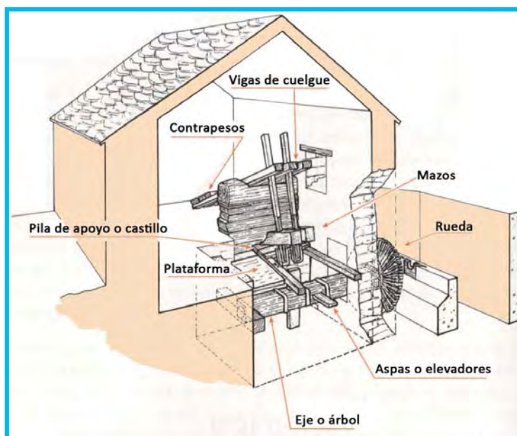
Esquema de un batán
