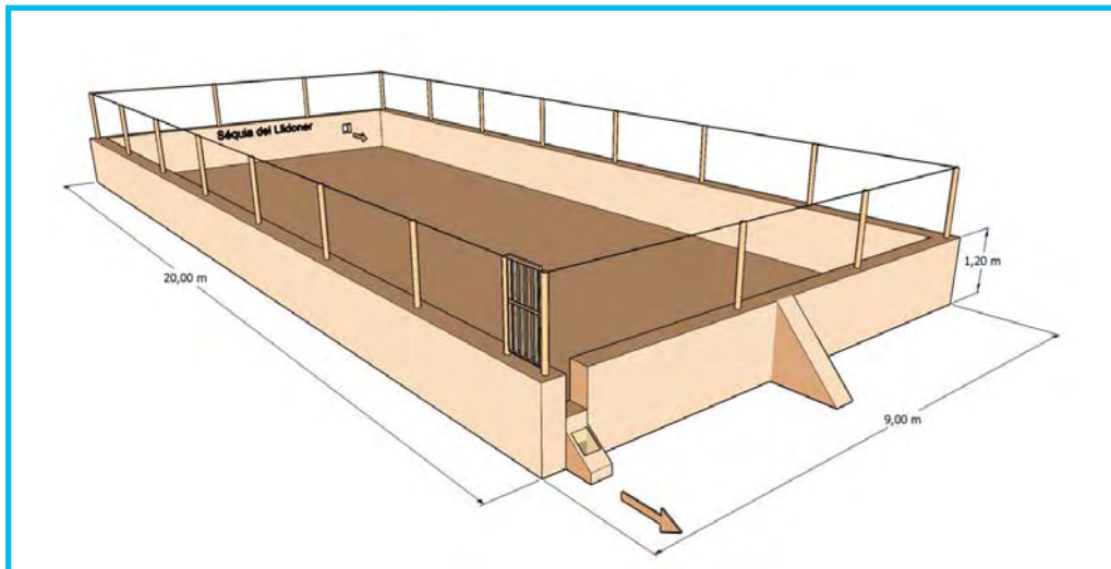
Esquema de una balsa, Balsa del Llidoner, Guadalest (Alicante)
