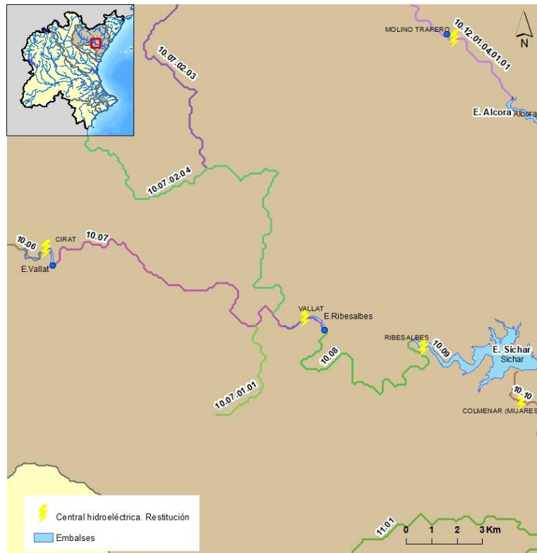
Figura 25. Detalle de las centrales hidroeléctricas en el tramo medio del río Mijares.
