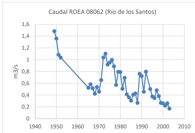
Figura 43. Evolución de caudal en la ROEA 08062 (Río de los Santos)
