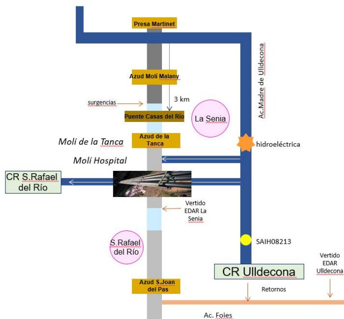
Figura 18. Esquema del río Sénia aguas abajo de la presa del Martinet hasta acequia Foies
