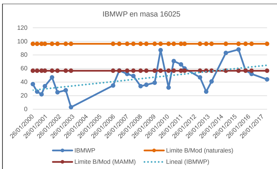
Figura 9. Evolución del indicador de macroinvertebrados (IBMWP) en el río Serpis: depuradora de Alcoy - Embalse de Beniarrés
