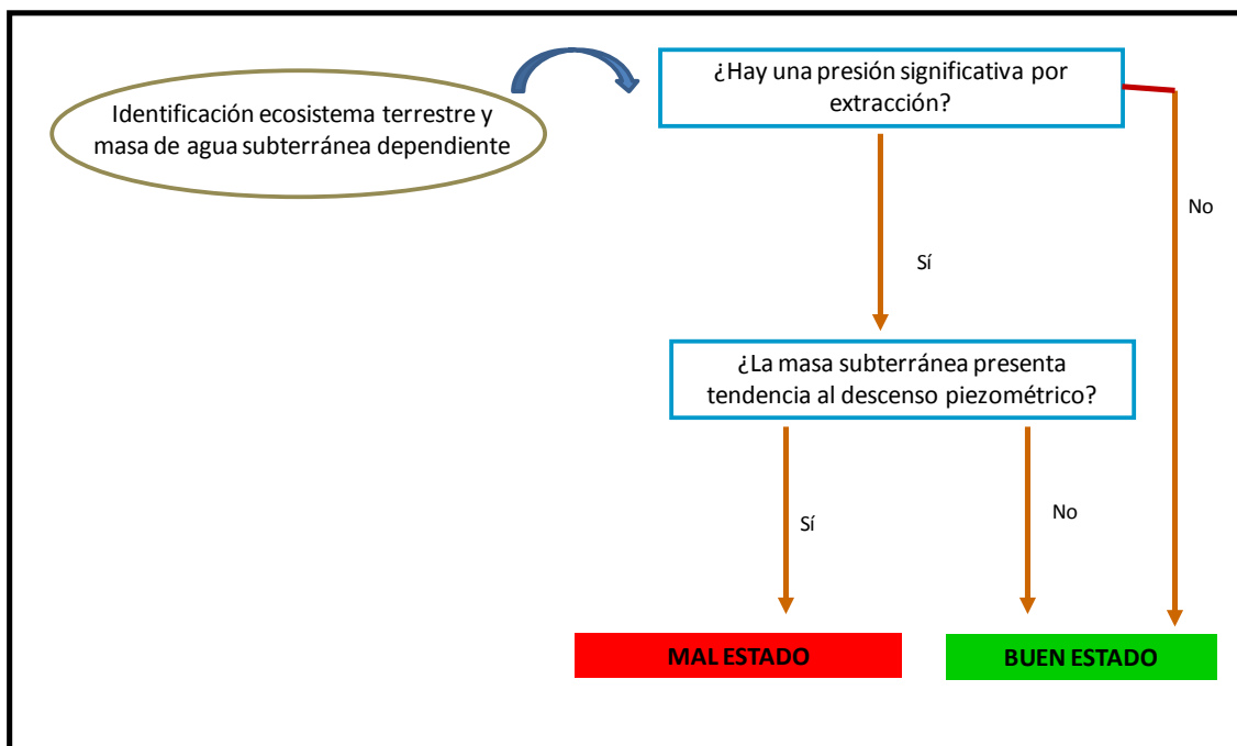
Figura 74. Esquema del procedimiento seguido en el test de ecosistemas terrestres dependientes de aguas subterráneas
