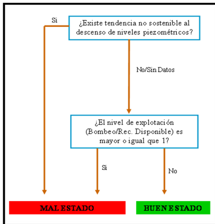
Figura 66. Esquema del procedimiento del test balance hídrico para evaluar el estado cuantitativo
