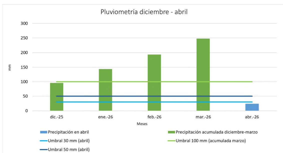
Figura 11 Pluviometría en la masa de agua subterránea 080-133 Requena – Utiel para la clasificación preliminar.
