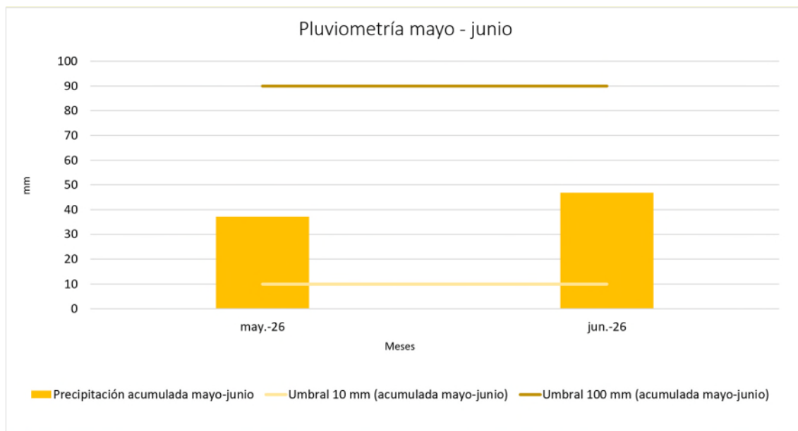
Figura 12 Pluviometría en la masa de agua subterránea 080-133 Requena – Utiel para la clasificación definitiva.
