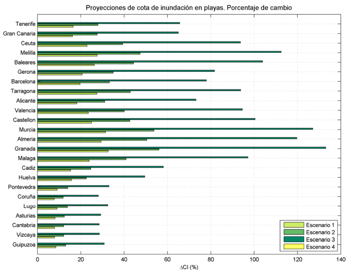
Figura 35. Porcentaje de cambio en la cota de inundación para los distintos escenarios de cambio climático por provincias. Fuente: IH Cantabria.
