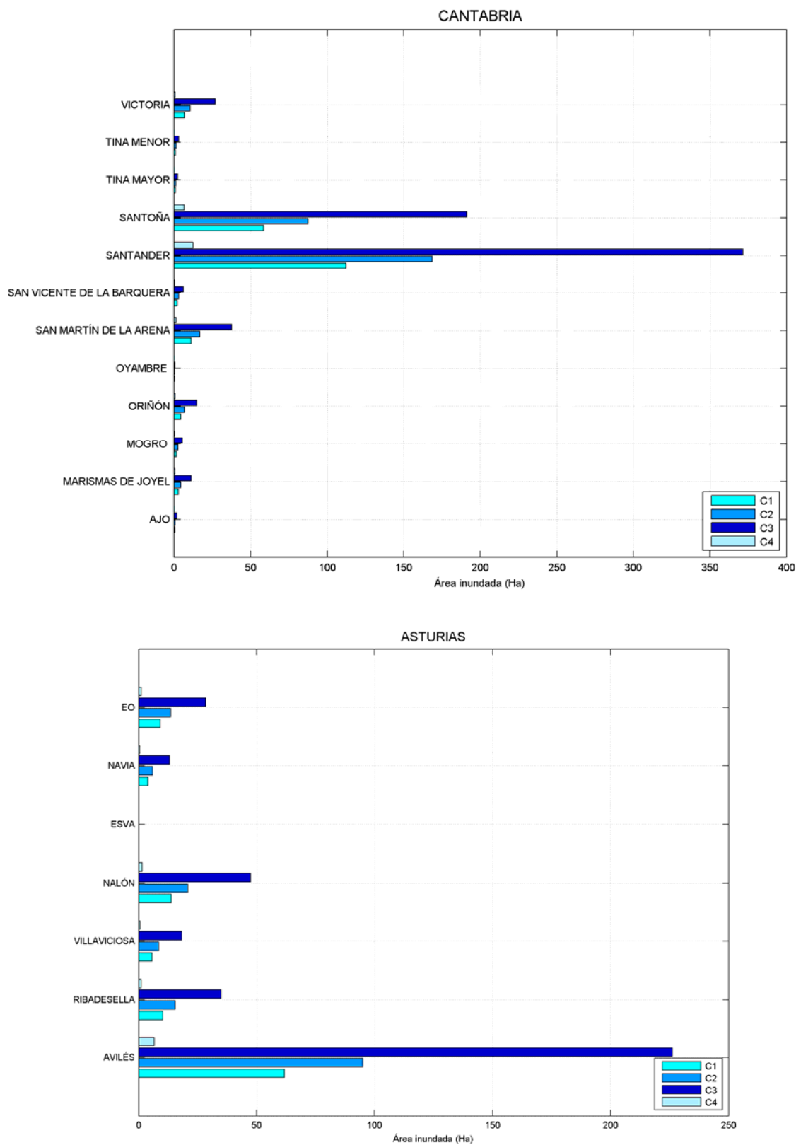
Figura 42. Pérdida potencial de humedales (Ha) debido a la subida del nivel del mar para los escenarios de cambio climático C1-C4 en el Cantábrico. Fuente: IH Cantabria.
