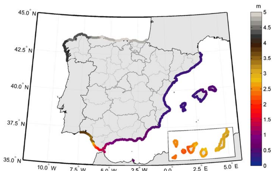
Figura 26. Rango de marea astronómica a lo largo del litoral español. Fuente: IH Cantabria
