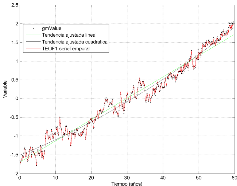
Figura 7. Tendencia y reconstrucción obtenida para el nivel medio del mar global. En rojo se representa la serie temporal del primer modo de la Trend-Eof mientras que los puntos negros (no coincidentes) representan el nivel medio global de la base de datos instrumental. Además, en verde y negro se representa las tendencias ajustadas, lineal y cuadrática, respectivamente. Fuente: IH Cantabria.
