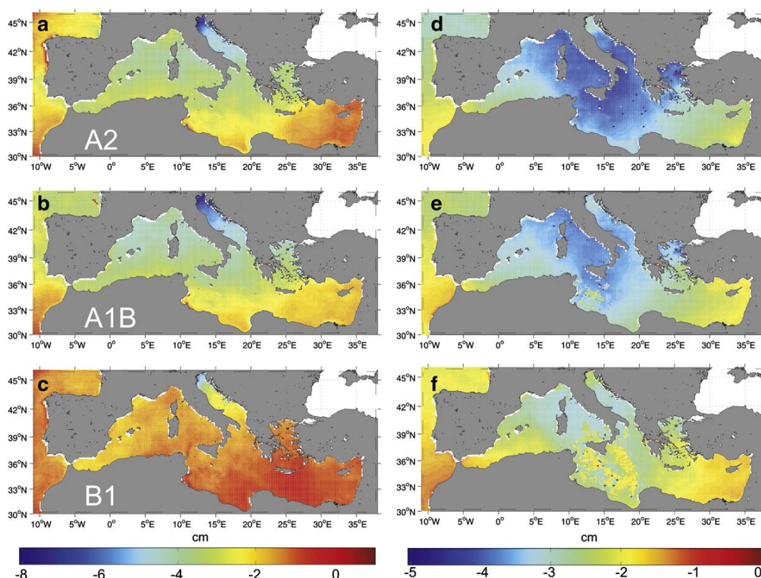
Figura 13. Cambios (cm) en el cuantil de marea meteorológica de 50 años de período de retorno en el período 2090-2099 para los escenarios A2, A1B y B1 con respecto al período 1990-1999 para sobreelevaciones positivas (a,b,c) y negativas (d,e,f). Fuente: Marcos et al. 2011.
