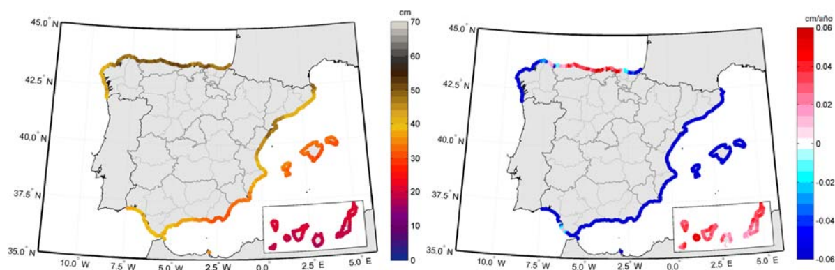
Figura 12. Marea meteorológica asociada a 50 años de período de retorno (izquierda) y tasa de cambio observada en los últimos 60 años en la marea meteorológica (derecha). Fuente: IH Cantabria.
