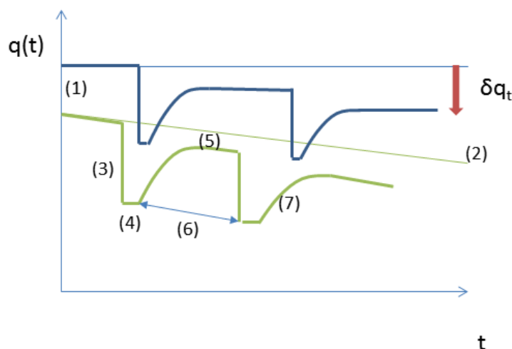
Figura 46. Esquema de la evolución de la producción de un activo natural sometido a cambio climático. Fuente: IH Cantabria.
