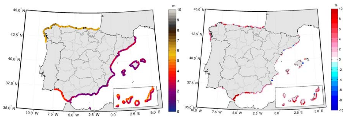
Figura 32. Cota de inundación asociada a 50 años de período de retorno en playas disipativas en el año 2040 (izquierda) y porcentaje de cambio en la cota de inundación respecto al siglo XX (derecha). Fuente: IH Cantabria.
