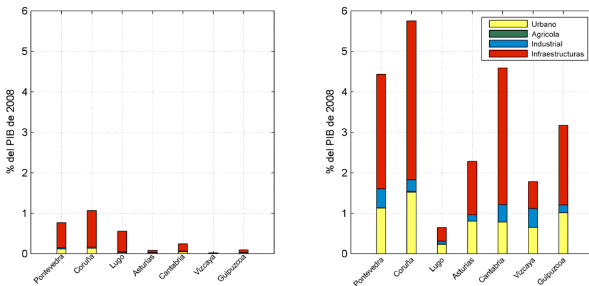
Figura 60. Valor medio anual del stock de capital afectado por inundación permanente (panel izquierdo) y valor del stock de capital afectado por eventos extremos de inundación (panel derecho) en términos de porcentaje sobre el PIB de 2008 en el año 2040. Valor actualizado al presente ( r=3\% ). Se considera evolución de la actividad económica en ausencia de medidas de adaptación. Fuente: IH Cantabria.
