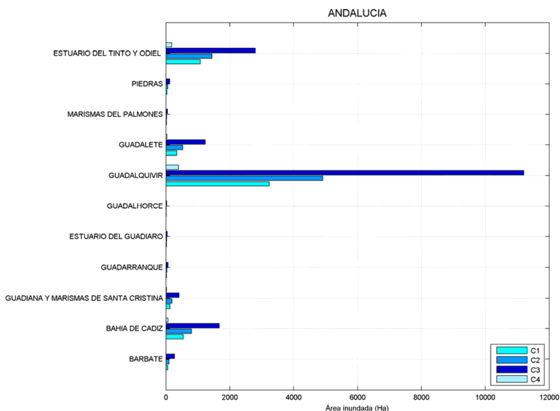
Figura 44. Pérdida de humedales (Ha) debido a la subida del nivel del mar para los escenarios de cambio climático C1-C4 en Andalucía. Fuente: IH Cantabria.
