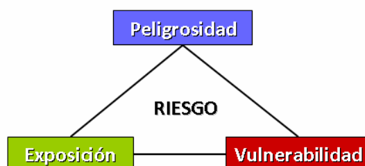
Figura 41. Esquema conceptual de la estimación del riesgo. Fuente: IH Cantabria.
