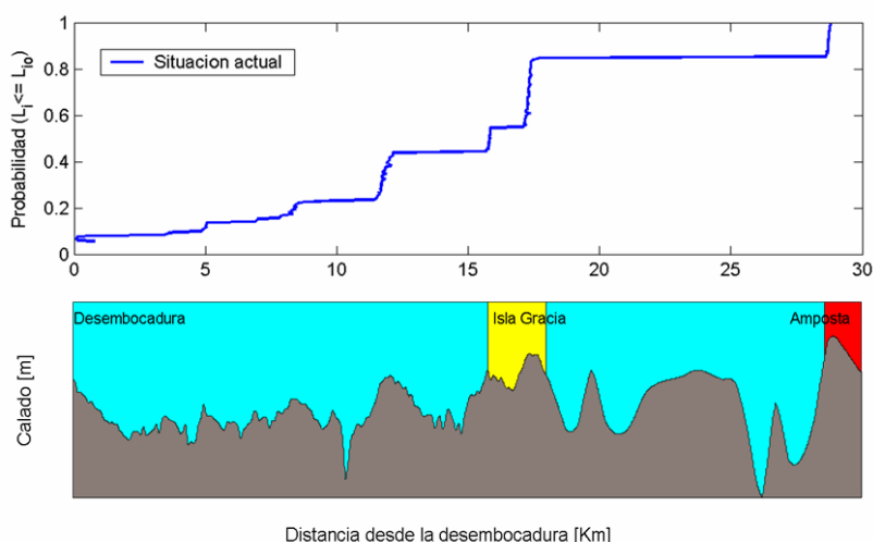
Figura 29. Régimen medio de avance de cuña salina en el Delta del Ebro para la situación actual. Fuente: Cambio Climático en el Delta del Ebro 2009.
