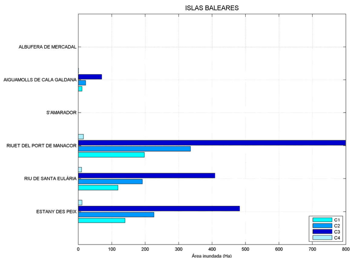
Figura 45. Pérdida de humedales (Ha) debido a la subida del nivel del mar para los escenarios de cambio climático C1-C4 en Mediterráneo español. Fuente: IH Cantabria
