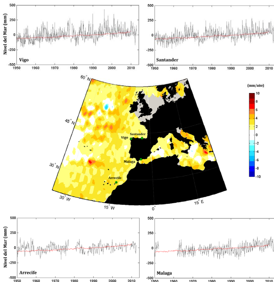
Figura 9. Mapa con los cambios estimados del nivel del mar durante el periodo 1993-2012 a partir de datos de altimetría de satélite. También se muestran los cambios relativos de nivel del mar medidos in-situ en diferentes estaciones de la costa española para el periodo 1950-2013 (línea gris) y para comparación con los registros locales se muestra el cambio global del nivel medio del mar (línea roja). Fuente: IH cantabria.
