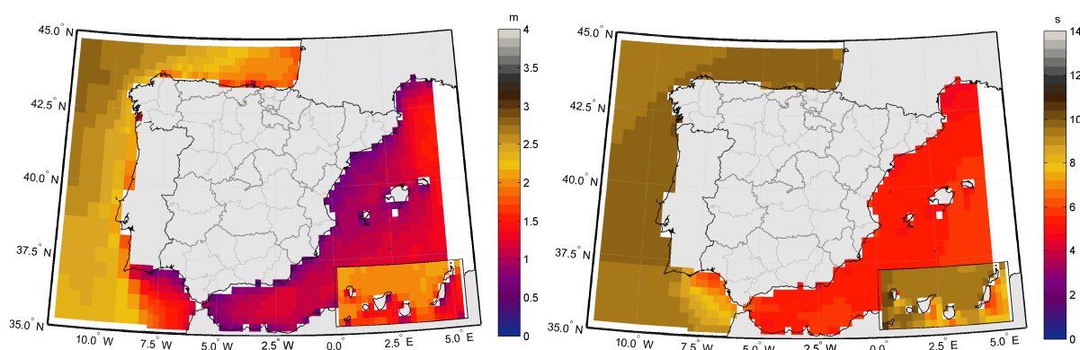
Figura 14. Altura de ola media anual en profundidades indefinidas en el entorno español (izquierda) y período de pico medio en profundidades indefinidas en el entorno español (derecha). Fuente: IH Cantabria.
