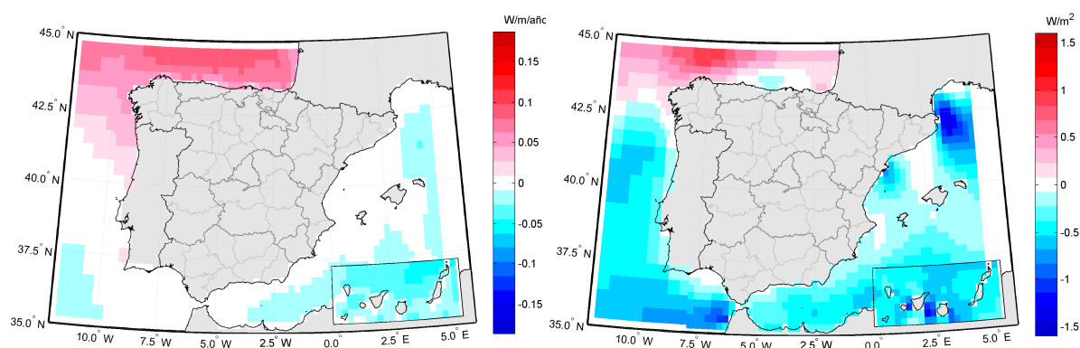
Figura 16. Tasa de cambios observados en el flujo medio de energía del oleaje (izquierda) y la potencia eólica (derecha) en los últimos 60 años. Fuente: IH Cantabria.
