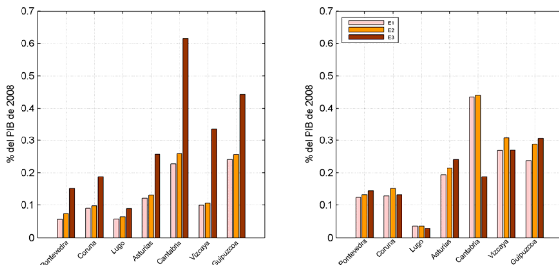
Figura 54. Valor en el año 2100 del PIB afectado en el caso de inundación permanente (panel izquierdo) y eventos extremos de inundación (panel derecho) en términos de porcentaje sobre el PIB de cada provincia en 2008 para los escenarios E1 a E3. Los valores han sido actualizados al presente ( r=3\% ). Hipótesis de crecimiento PIB (0%). Fuente: IH Cantabria.
