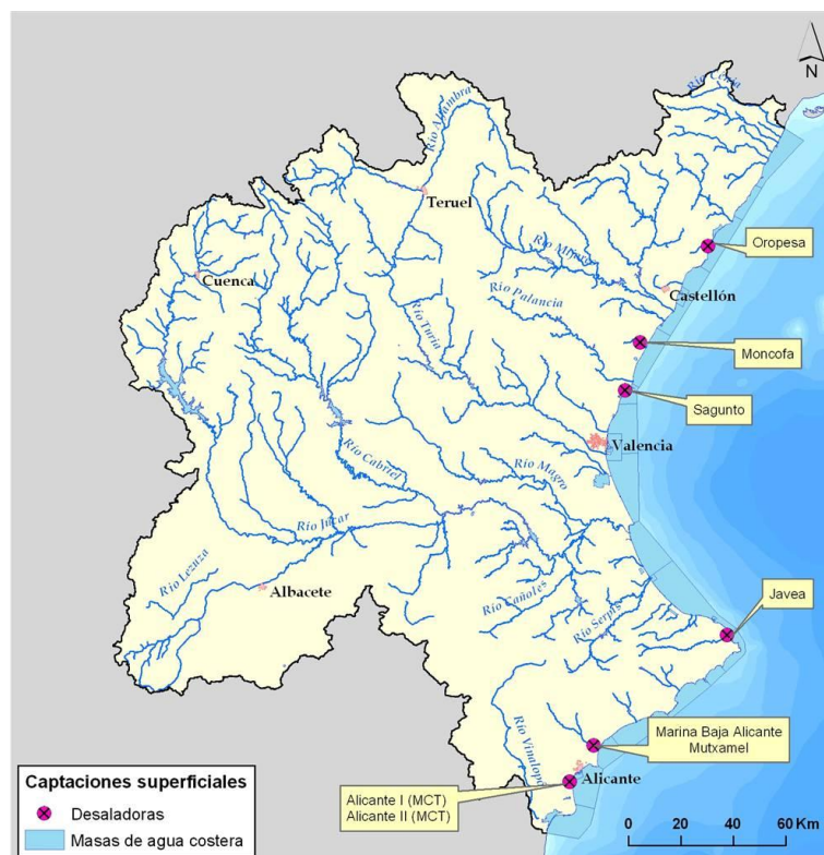
Figura 3. Captaciones de agua costera para abastecimiento urbano en DHJ.
