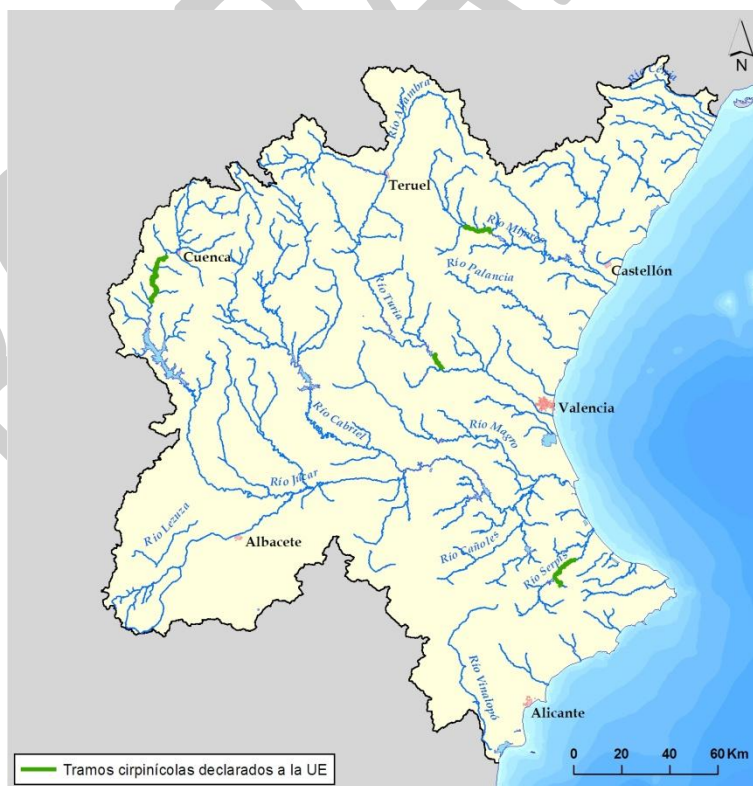
Figura 5. Zonas de producción de peces.
