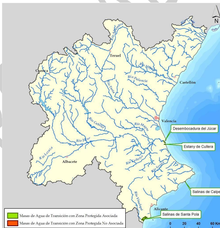
Figura 22. Masas de agua superficial tipo transición con zona protegida asociada
