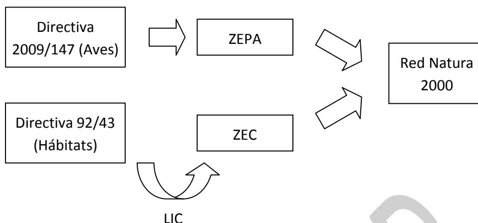
Figura 12. Estructura de la red Natura 2000
