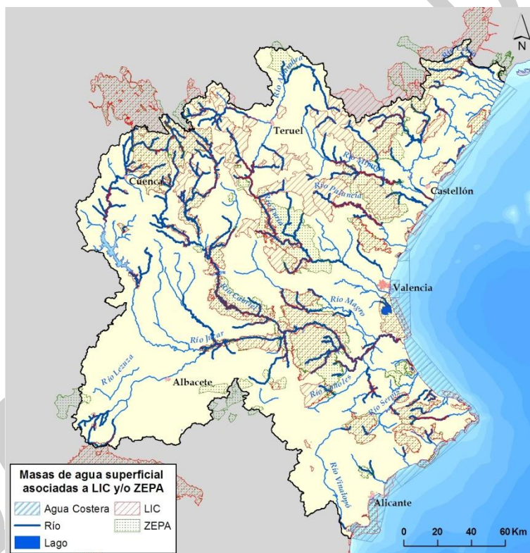
Figura 13. Masas de agua superficial asociadas a LIC y/o ZEPA. LIC y ZEPA asociadas al medio acuático en la DHJ.
