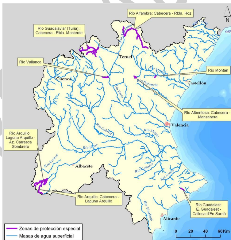
Figura 17. Zonas de protección especial
