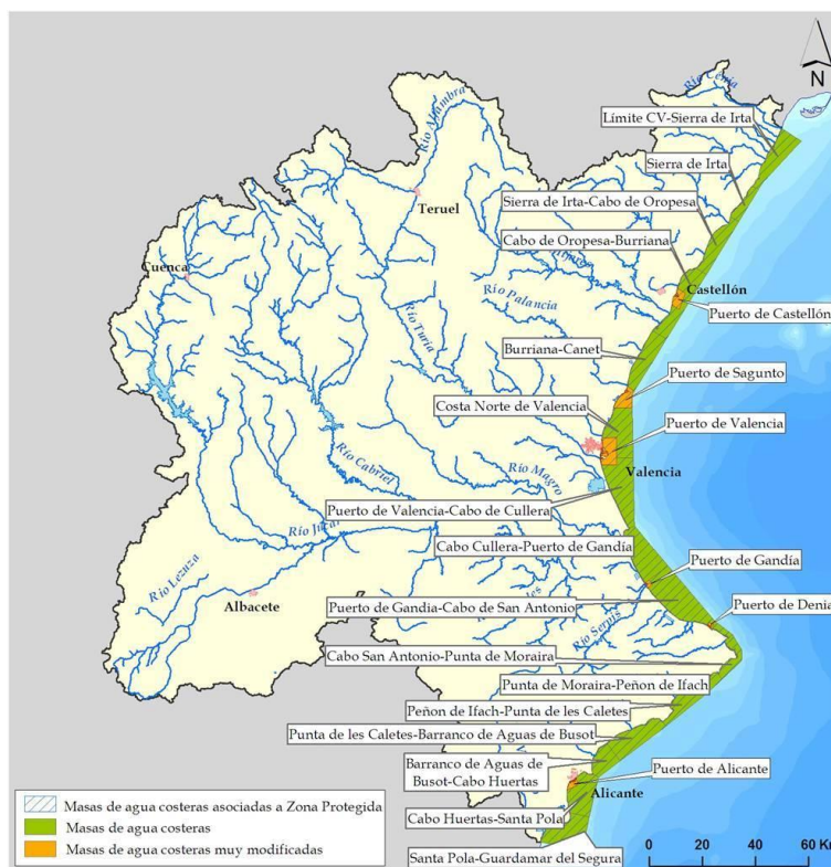
Figura 23. Masas de agua superficial costera con zona protegida asociada
