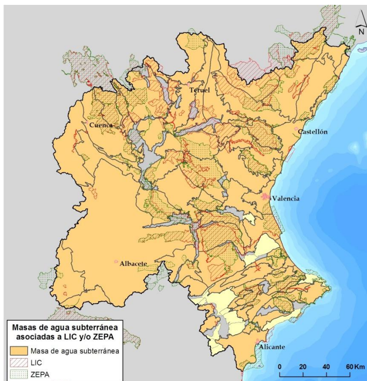
Figura 14. Masas de agua subterránea asociadas a LIC y/o ZEPA. LIC y ZEPA asociadas al medio acuático en la DHJ.
