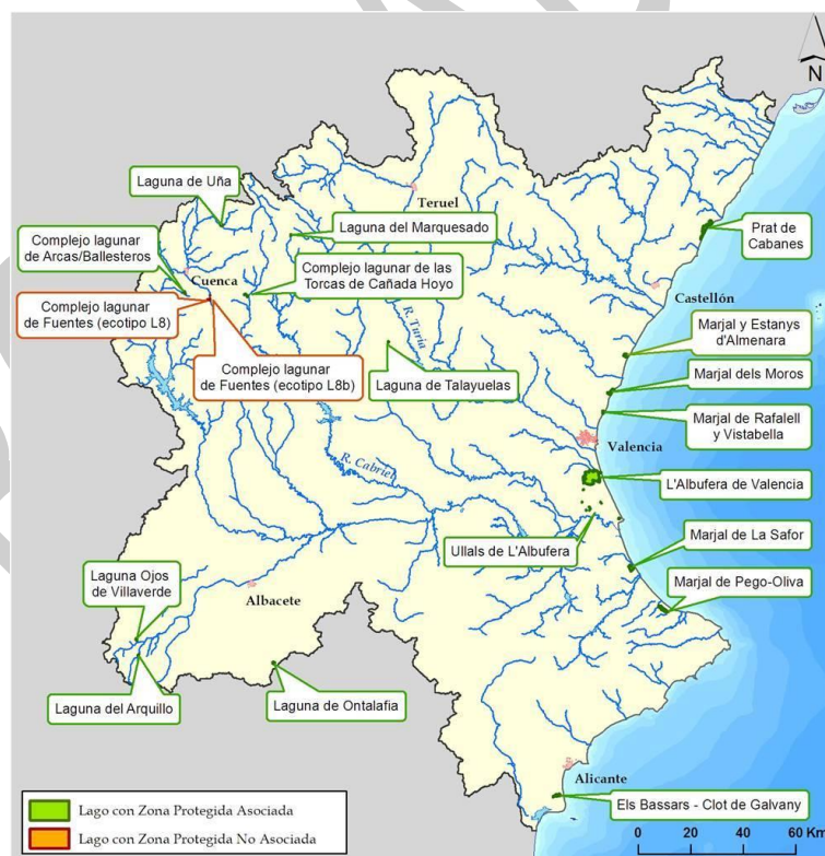
Figura 21. Masas de Agua superficial tipo lago con zona protegida asociada
