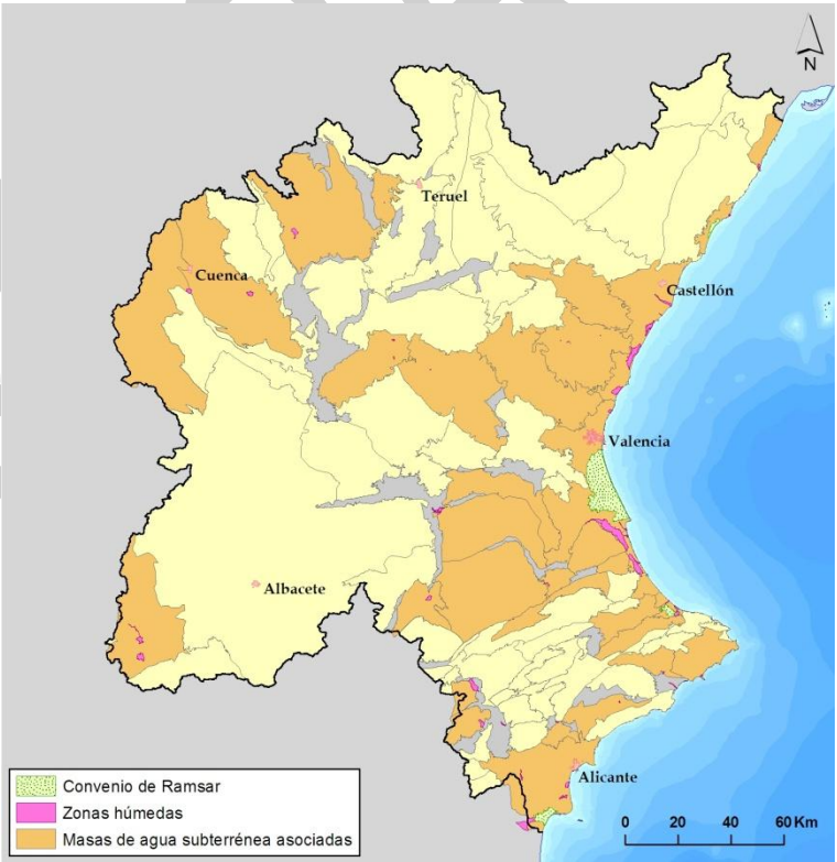
Figura 19. Masas de agua subterránea asociadas a las zonas húmedas
