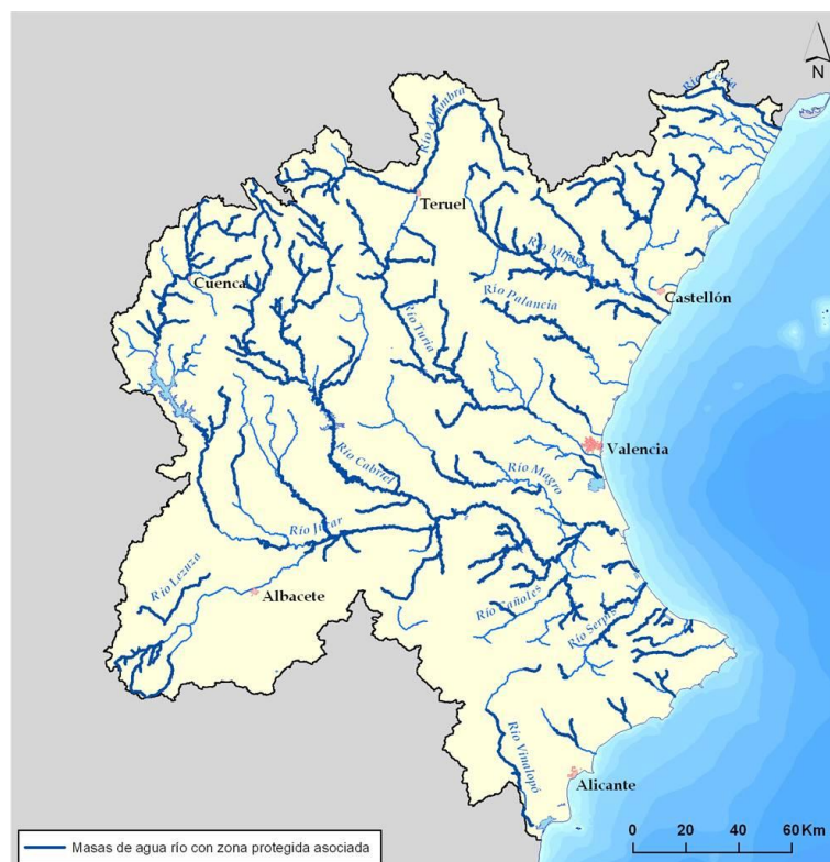
Figura 20. Masas de Agua superficial tipo río con zona protegida asociada
