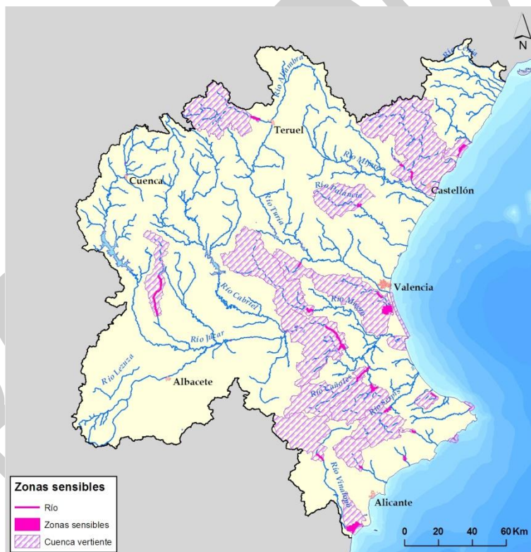
Figura 11. Zonas sensibles en aguas continentales y marinas.
