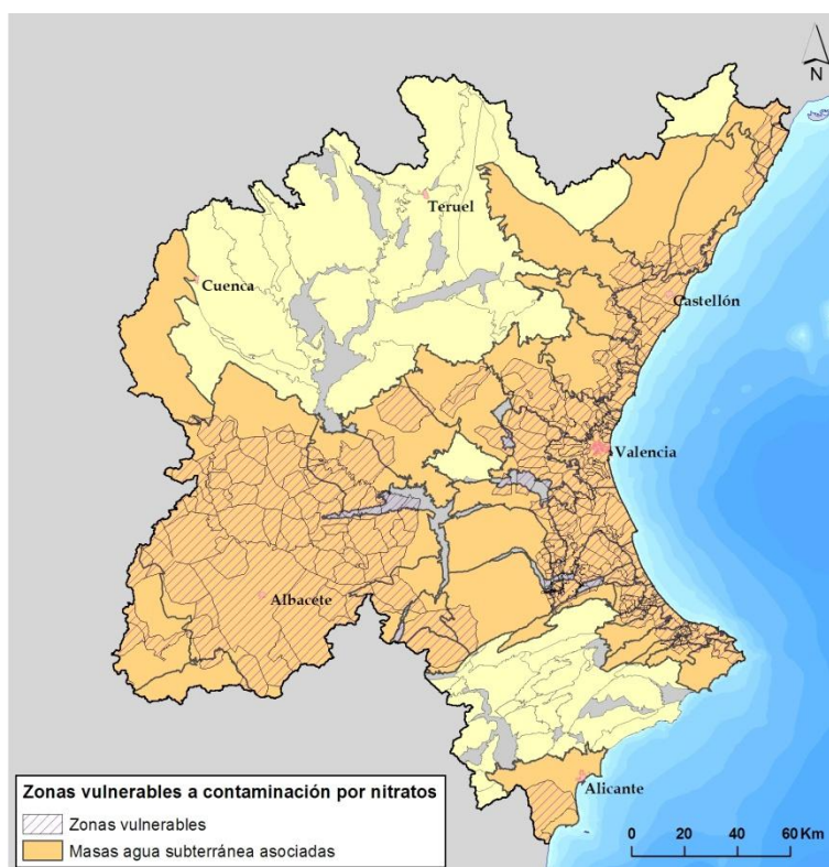
Figura 8. Zonas vulnerables a la contaminación por nitratos.
