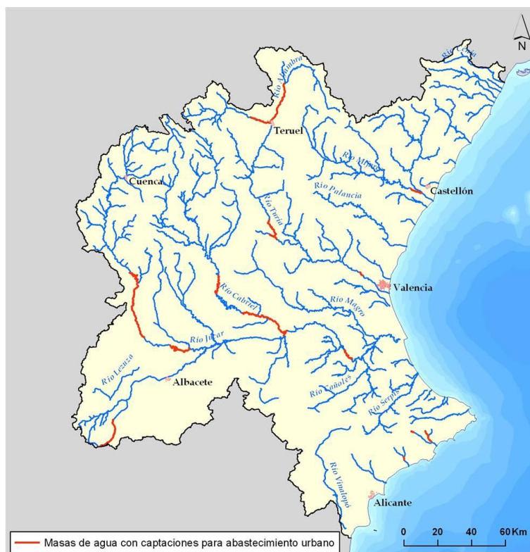
Figura 1. Captaciones de agua superficial para abastecimiento urbano en la DHJ.
