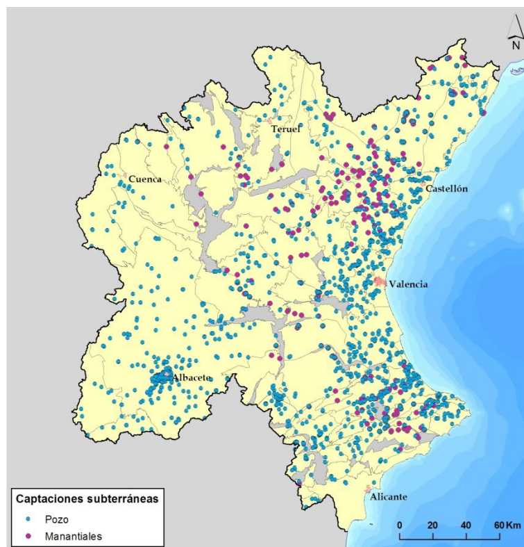
Figura 4. Captaciones de agua subterránea para abastecimiento urbano en DHJ.
