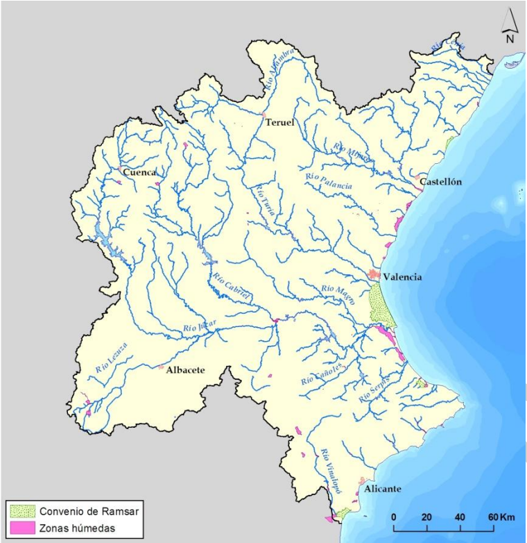
Figura 18. Zonas húmedas
