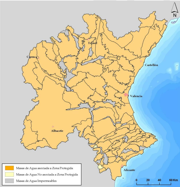
Figura 24. Masas de agua subterránea con zona protegida asociada
