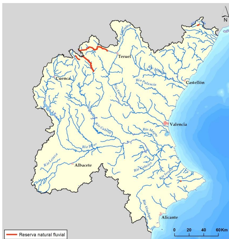
Figura 16. Tramos de río propuestos para ser declarados como reservas naturales fluviales
