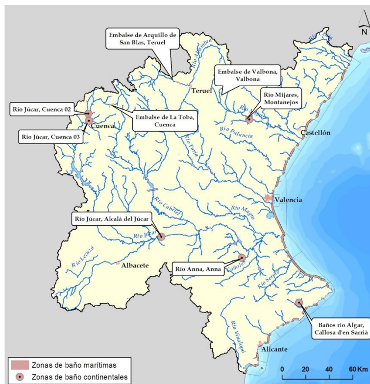
Figura 7. Zonas de baño en aguas continentales y marinas
