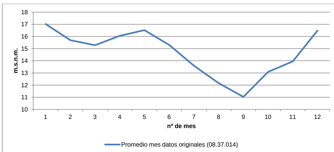
Figura 73. Promedio mensual de los datos originales del piezómetro de Pego (08.37.014).
