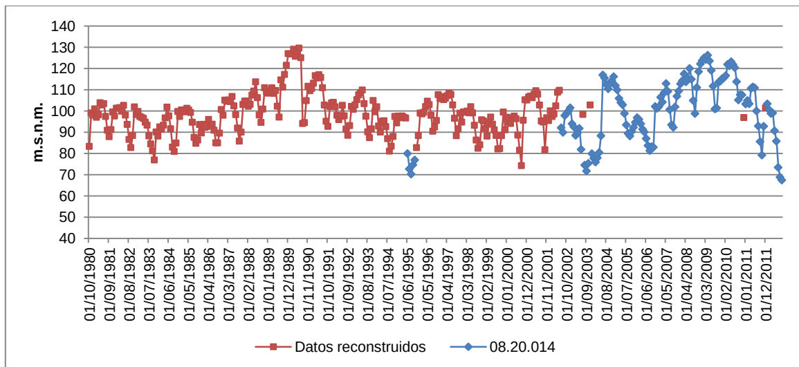
Figura 81. Serie de piezometría mensual completada del piezómetro de Sagunto (08.20.014).
