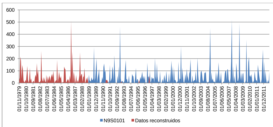
Figura 36. Serie de precipitación mensual completada (mm) del pluviómetro Beniarrés (N9S0101).
