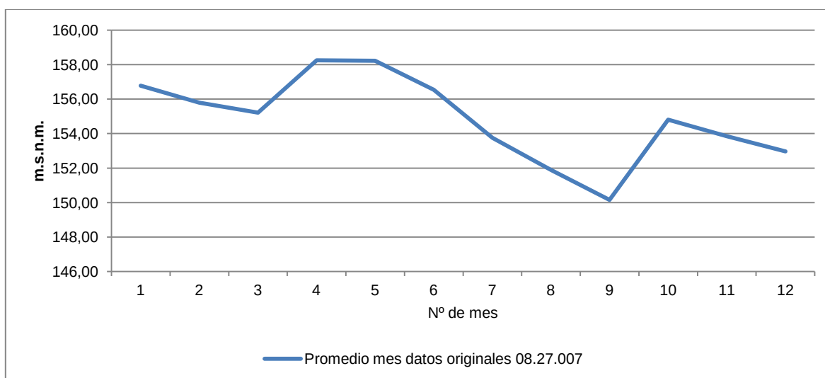
Figura 68. Promedio mensual de los datos originales del piezómetro de Montesa (08.28.007).
