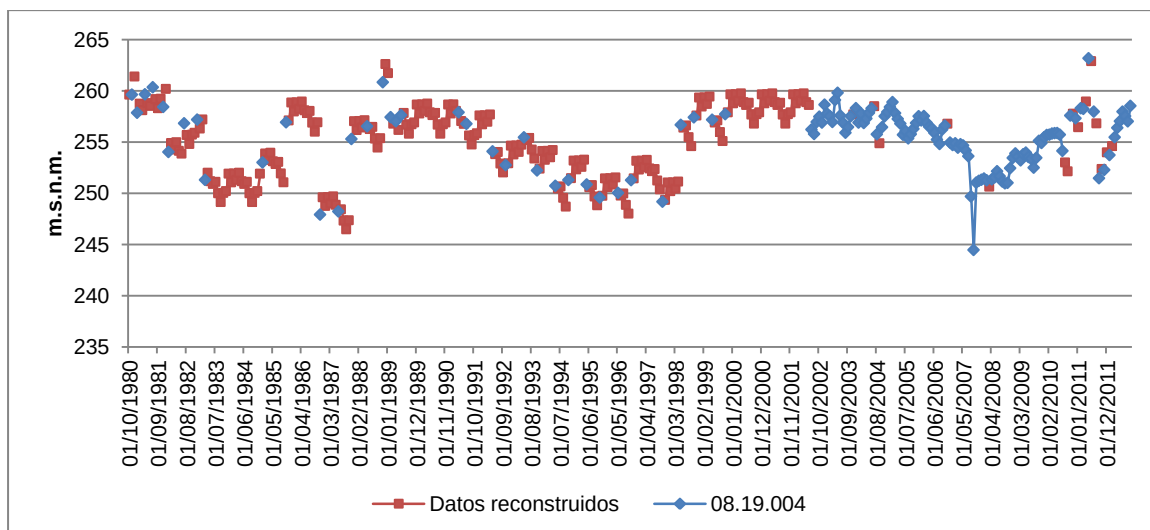
Figura 84. Serie de piezometría mensual completada del piezómetro de Lliria (08.19.004).
