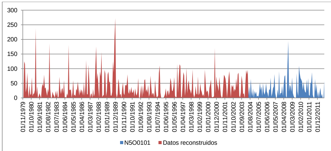
Figura 49. Serie de precipitación mensual completada (mm) del pluviómetro Villatoya (N5O0101).
