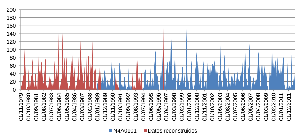
Figura 23. Serie de precipitación mensual completada (mm) del pluviómetro Aforo en Cuenca (N4A0101)
