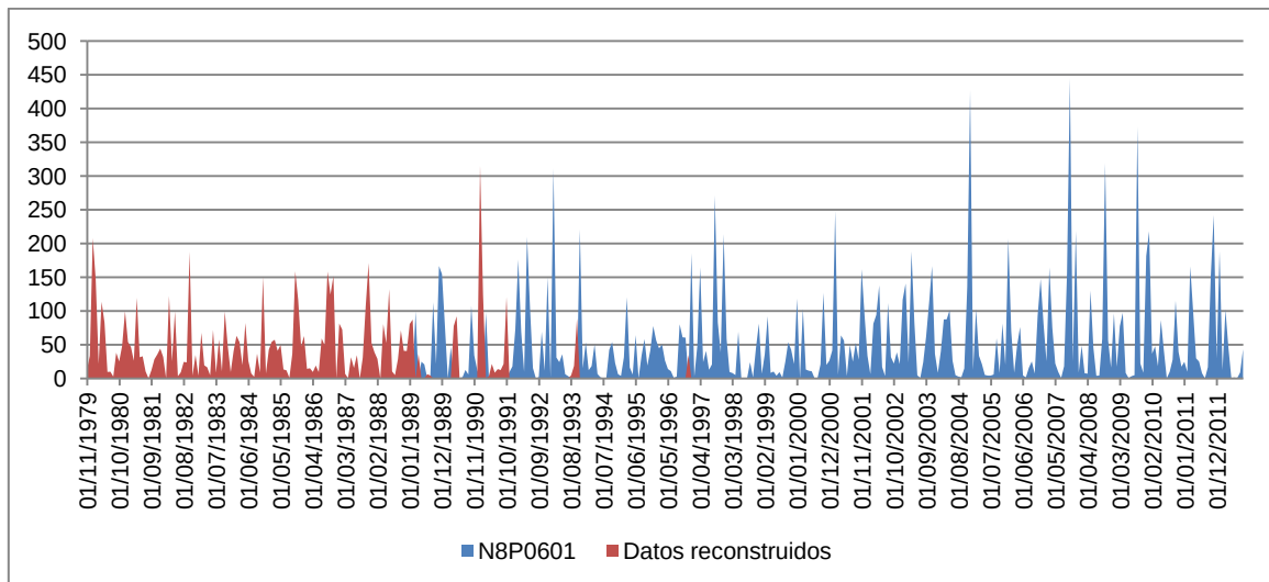
Figura 41. Serie de precipitación mensual completada (mm) del pluviómetro Abdet (N8P0601).
