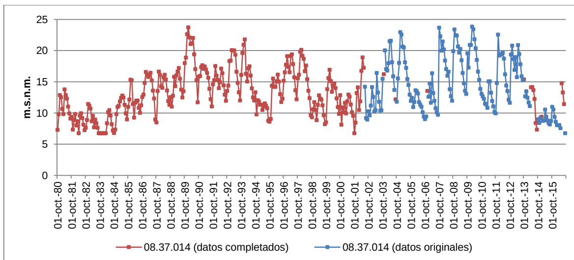
Figura 76. Serie de piezometría mensual completa del piezómetro de Pego (08.37.014).
