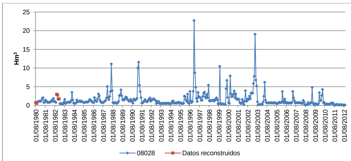
Figura 61. Serie de aportación mensual completada para la estación de aforo de Villalba Alta (08028).
