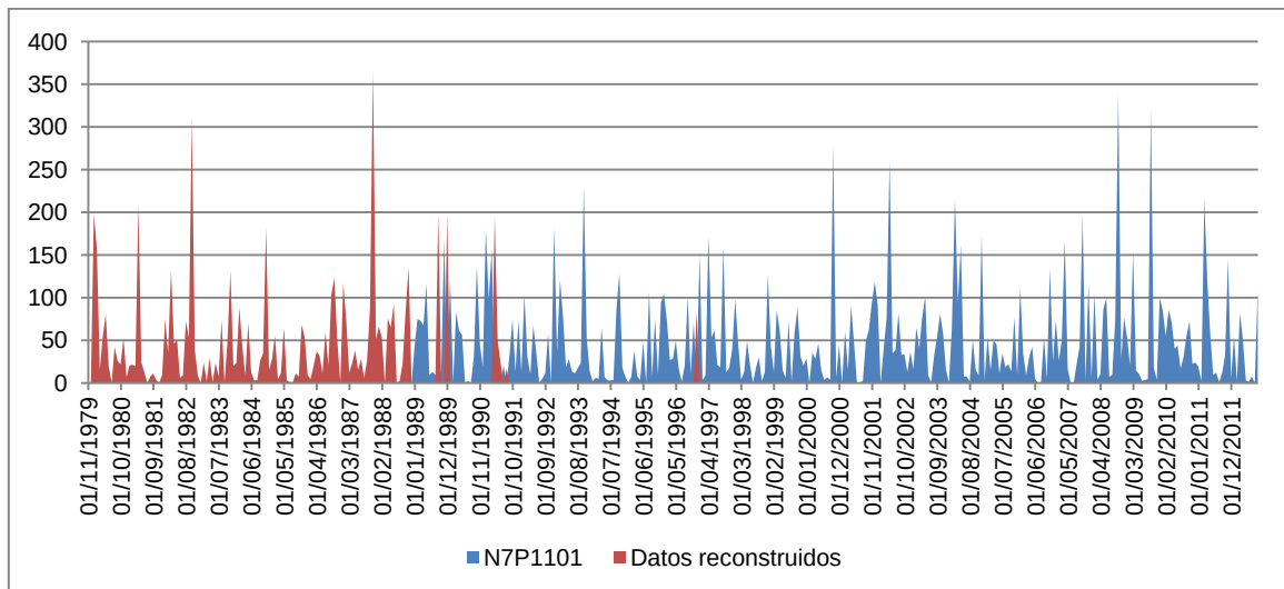
Figura 50. Serie de precipitación mensual completada (mm) del pluviómetro Sierra Ave (N7P1101).
