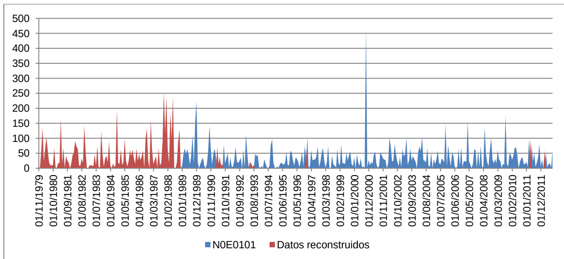
Figura 10. Serie de precipitación mensual completada (mm) del pluviómetro Embalse de Regajo (N0E0101).
