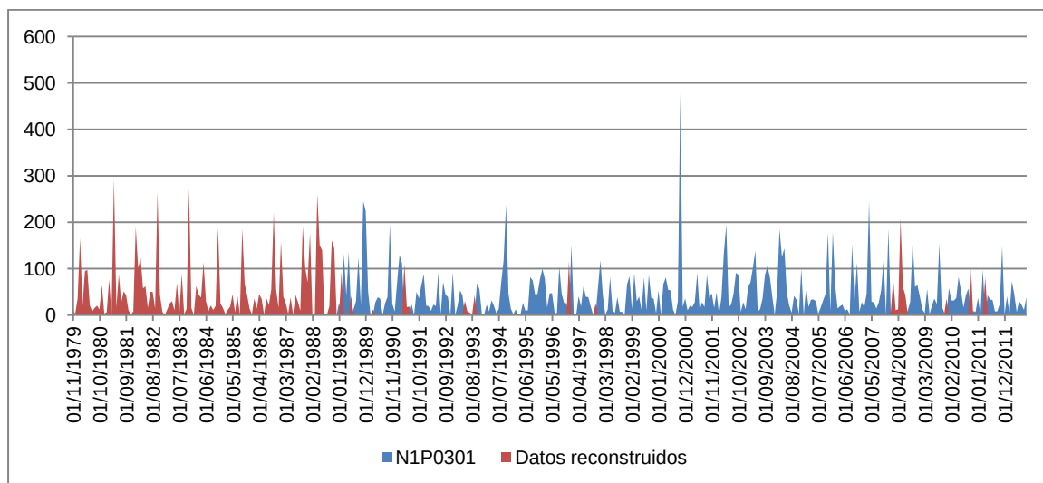
Figura 2. Serie de precipitación mensual completada (mm) del pluviómetro Xert (N1P0301).
