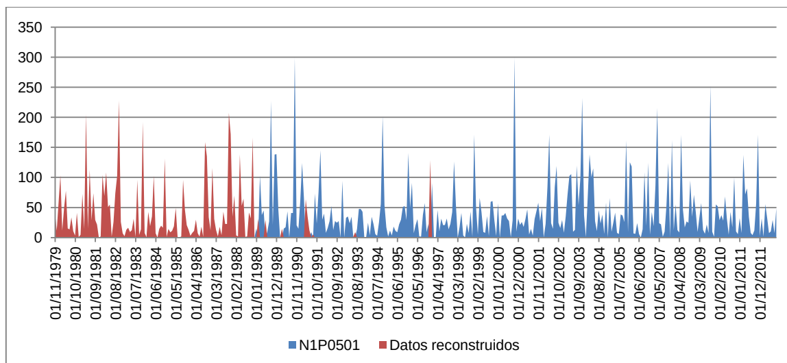
Figura 4. Serie de precipitación mensual completada (mm) del pluviómetro Alcalá de Chivert (N1P0501).
