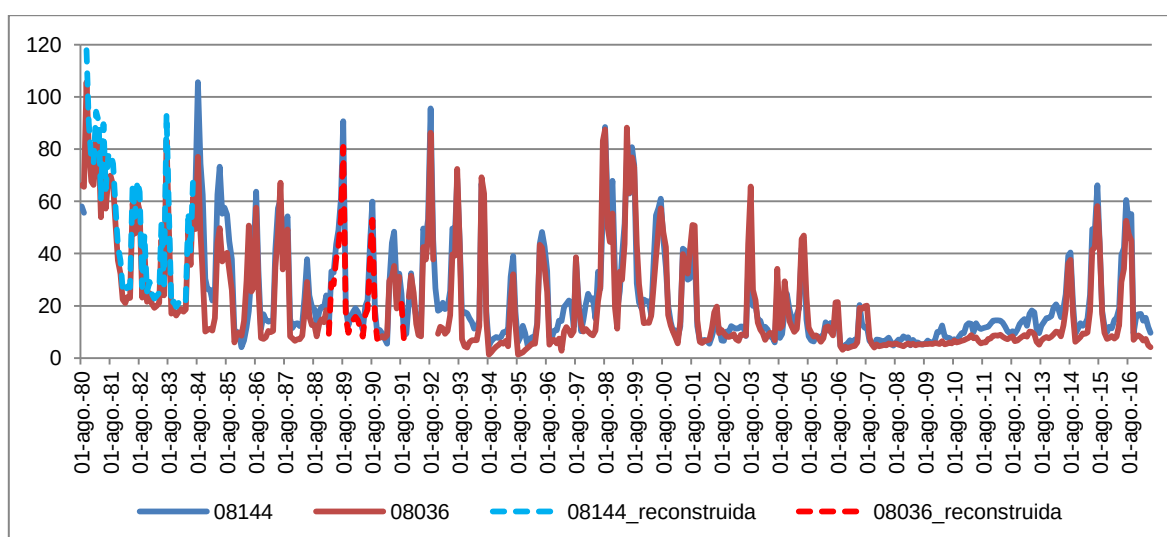
Figura 59. Correlación entre las estaciones 08144 y 08036.
