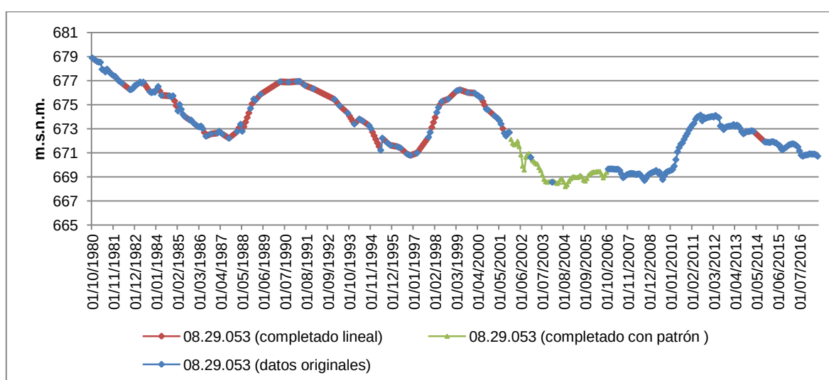
Figura 71. Serie de piezometría mensual completa del piezómetro de Cenizate (08.29.053).
