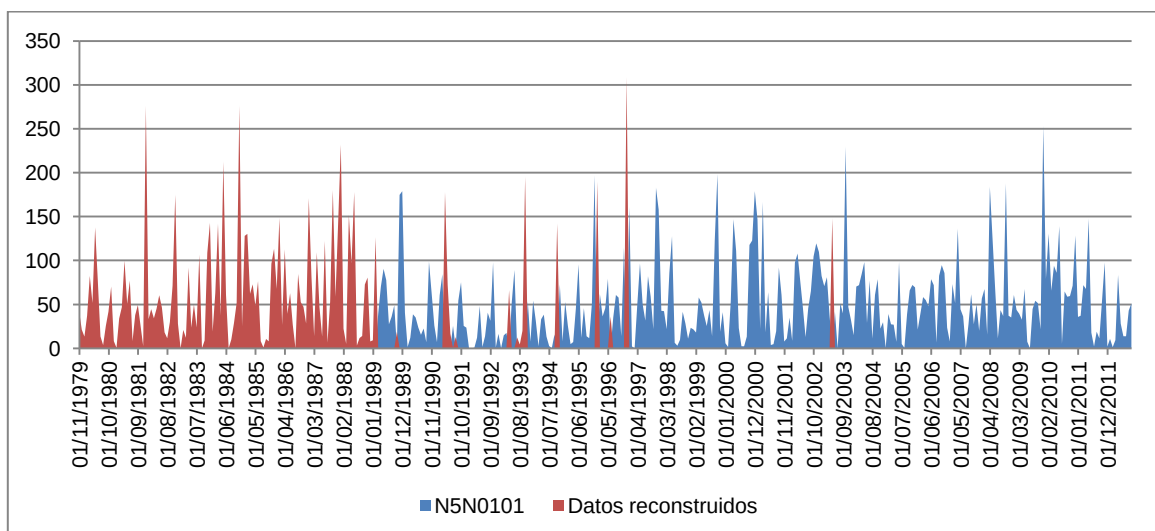
Figura 24. Serie de precipitación mensual completada (mm) del Pluvionivómetro Laguna del Marquesado (N5N0101).
