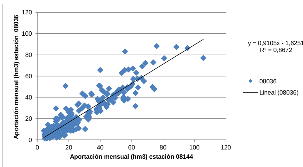
Figura 59. Correlación entre las estaciones 08144 y 08036.
