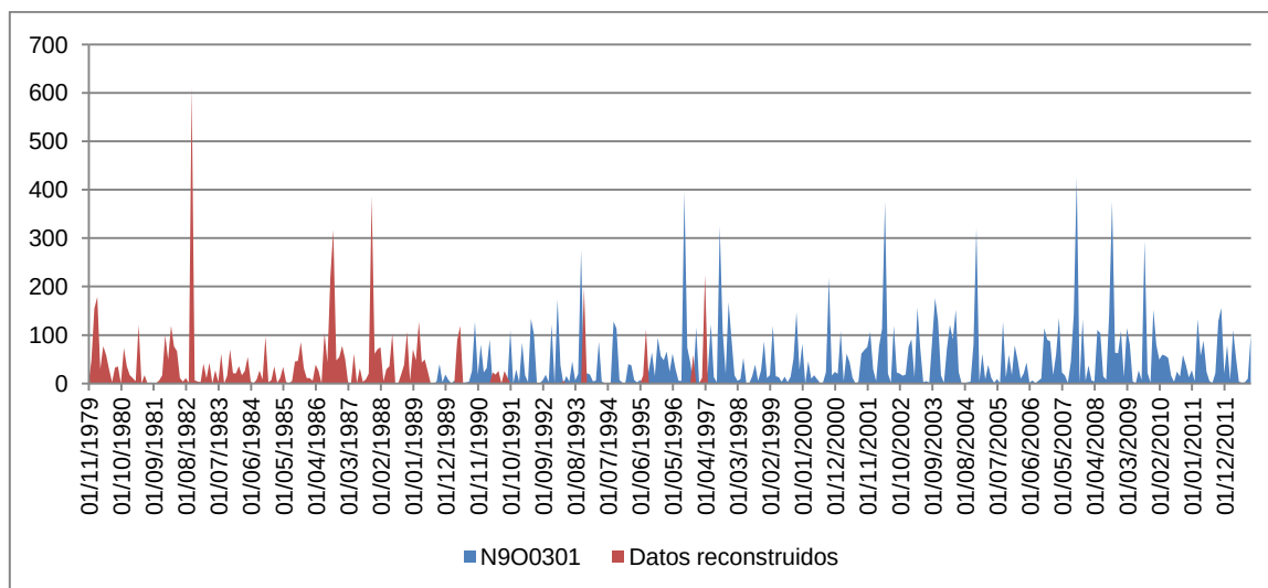
Figura 35. Serie de precipitación mensual completada (mm) del pluviómetro Marco en río Vernissa (N9O0301).
