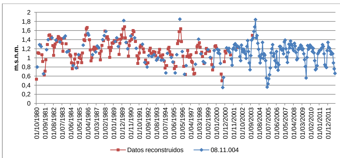
Figura 77. Serie de piezometría mensual completada del piezómetro de Cabanes (08.11.004).
