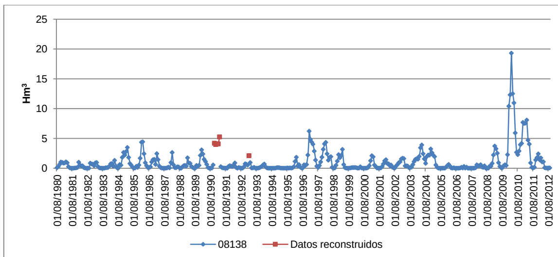
Figura 64. Serie de aportación mensual completada para la estación de aforo de Balazote (08138).
