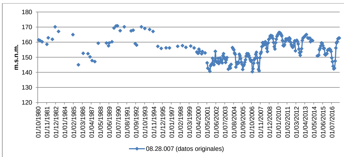
Figura 67. Serie de piezometría mensual original del piezómetro de Montesa (08.28.007).
