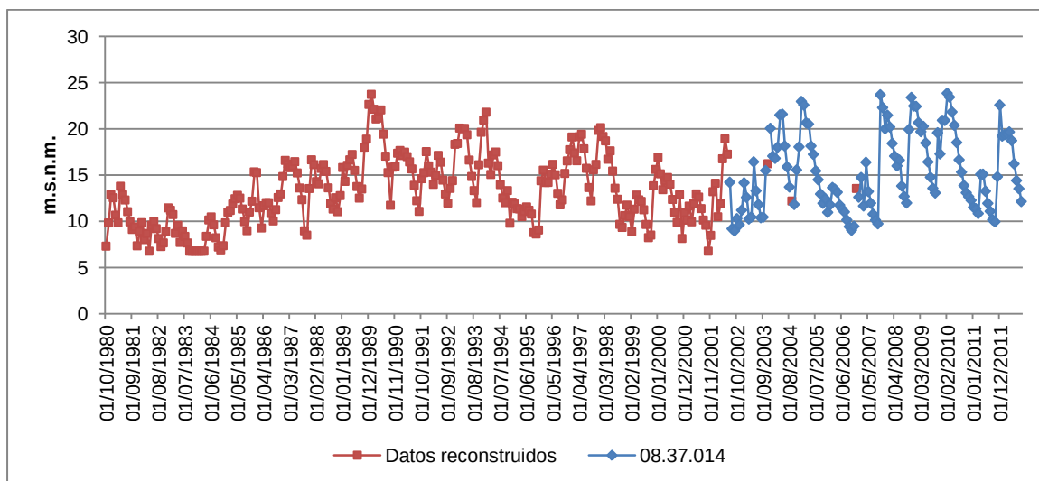
Figura 91. Serie de piezometría mensual completada del piezómetro de Pego (08.37.014).
