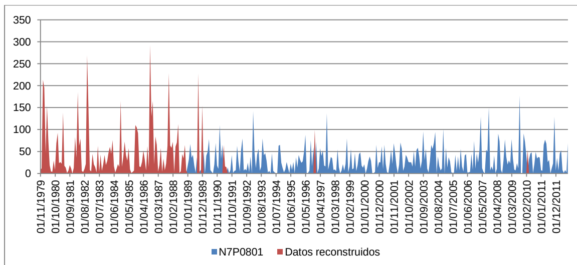
Figura 52. Serie de precipitación mensual completada (mm) del pluviómetro Font de la Figuera (N7P0801).
