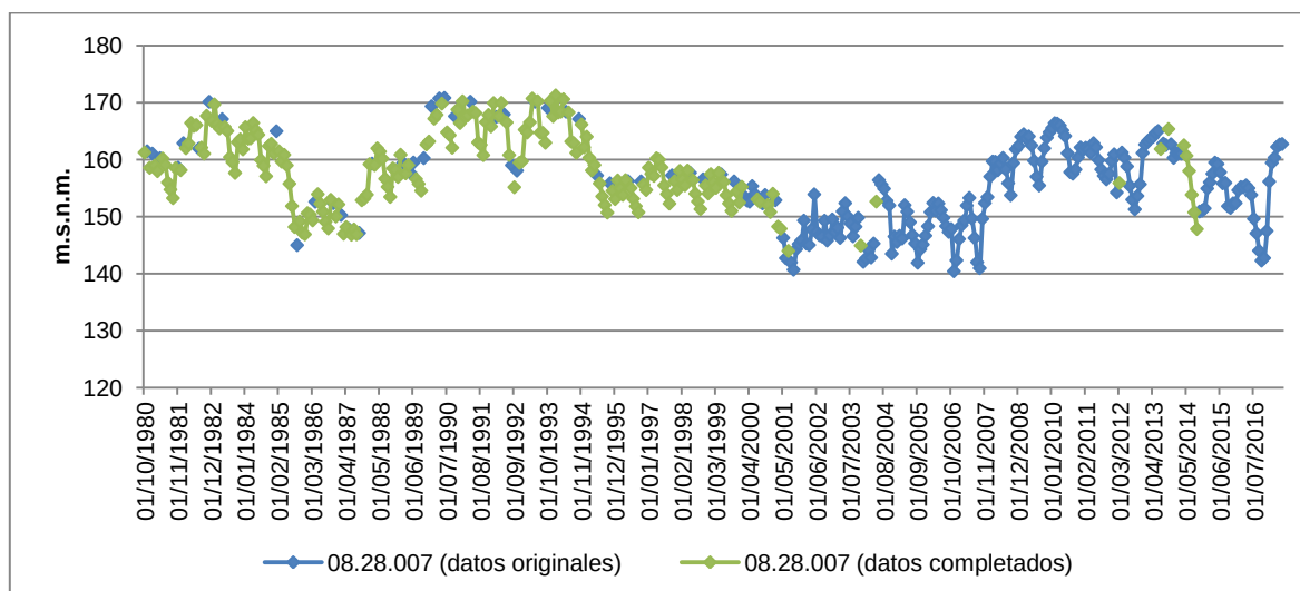
Figura 70. Serie de piezometría mensual completa del piezómetro de Montesa (08.28.007).
