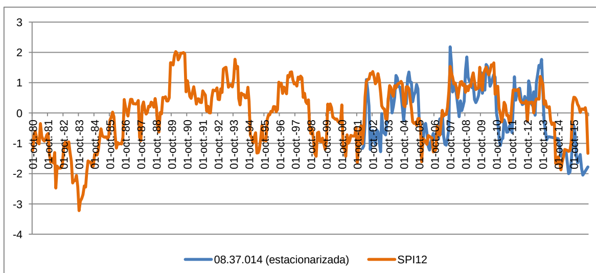
Figura 74. Datos estacionarizados para la serie del piezómetro de Pego (08.37.014) y valores del SPI12.
