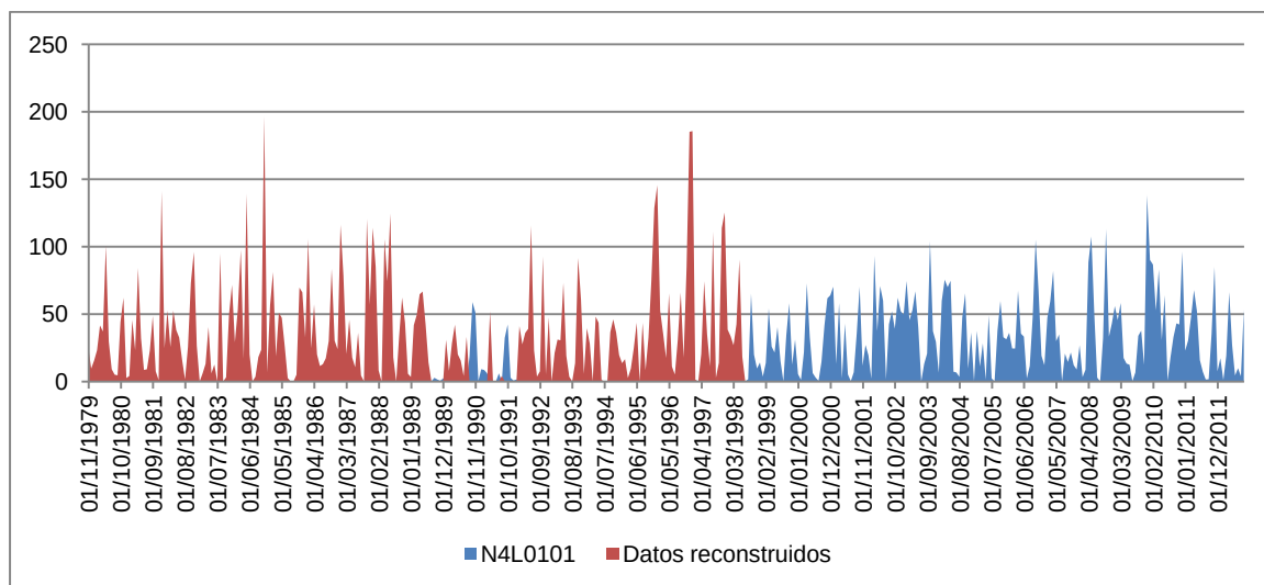
Figura 26. Serie de precipitación mensual completada (mm) del pluviómetro Belmontejo (N4L0101).
