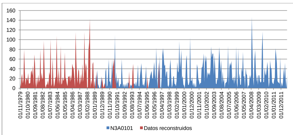
Figura 12. Serie de precipitación mensual completada (mm) del pluviómetro Aforo en Villalba Alta (N3A0101).
