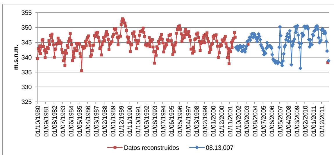
Figura 80. Serie de piezometría mensual completada del piezómetro de Eslida (08.13.007).
