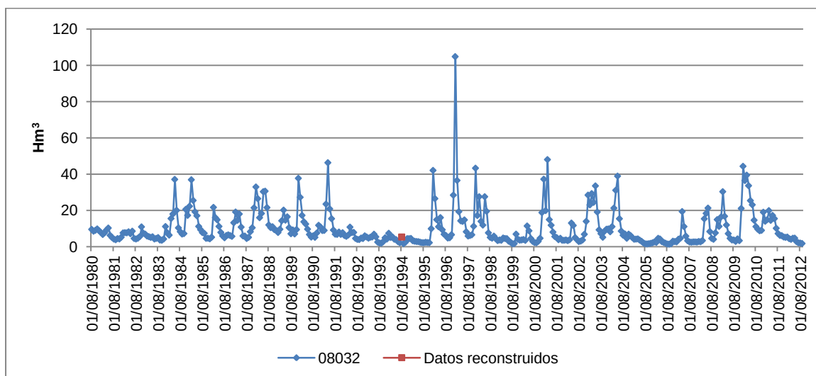
Figura 62. Serie de aportación mensual completada para la estación de aforo de Cuenca (08032).
