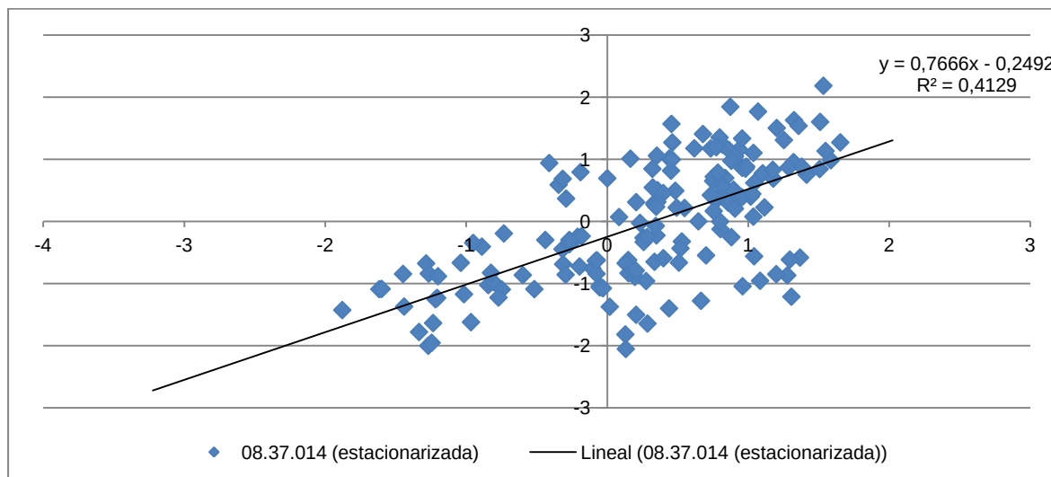
Figura 75. Correlación entre la serie estacionarizada del piezómetro de Pego y los valores del SPI12.
