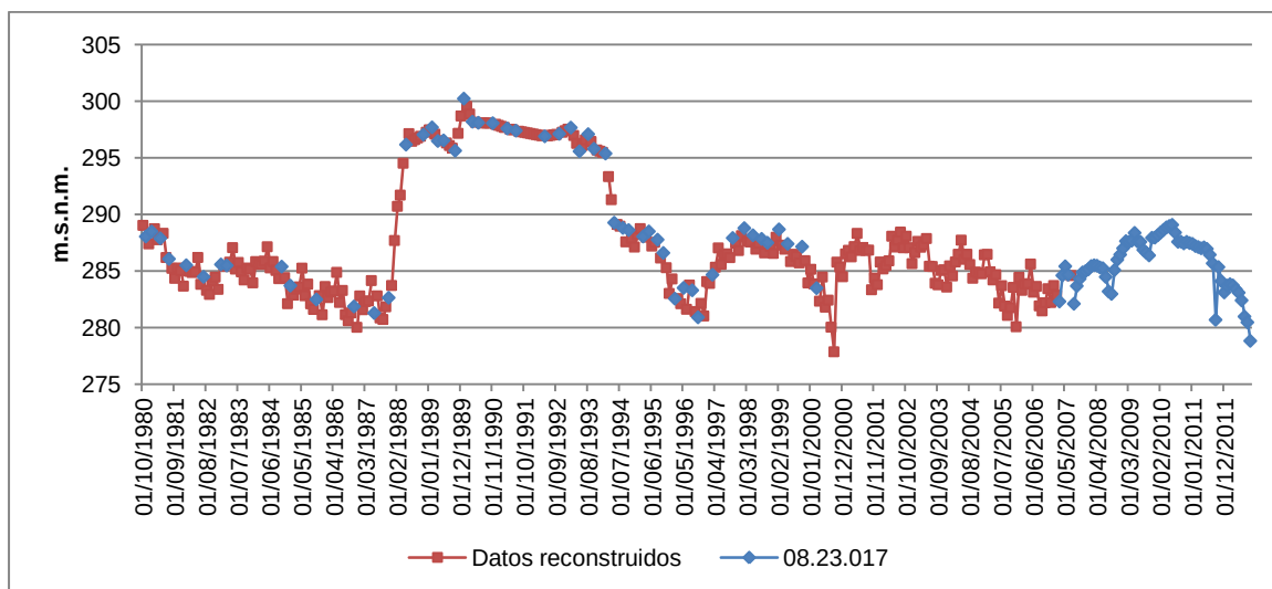
Figura 85. Serie de piezometría mensual completada del piezómetro de Chiva (08.23.017).
