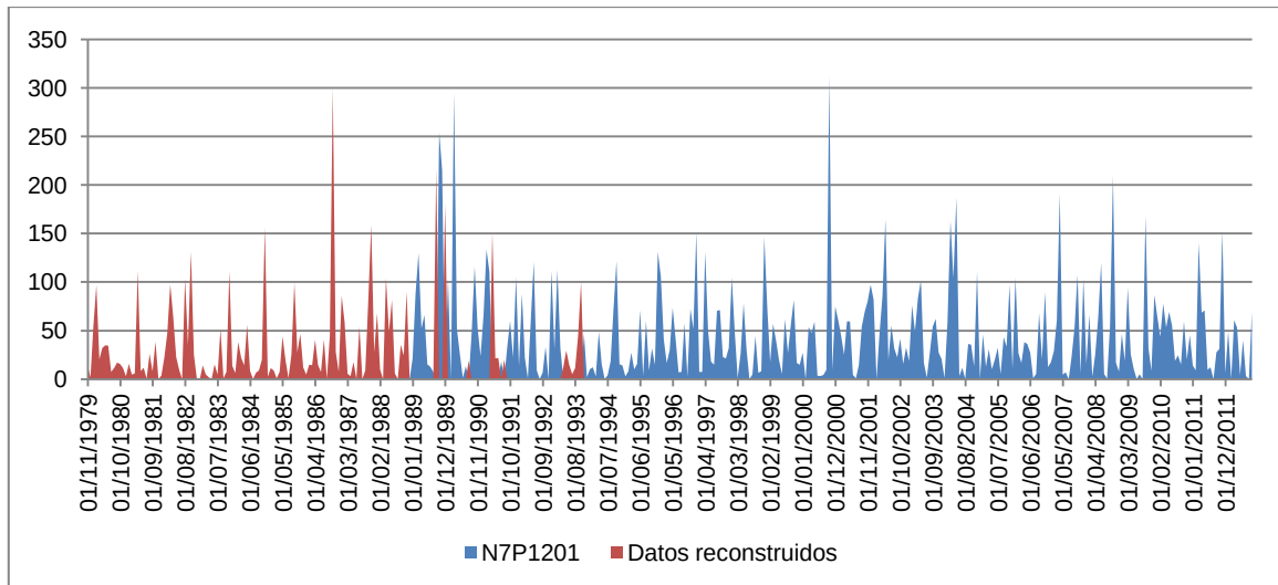
Figura 22. Serie de precipitación mensual completada (mm) del pluviómetro Siete Aguas (N7P1201).
