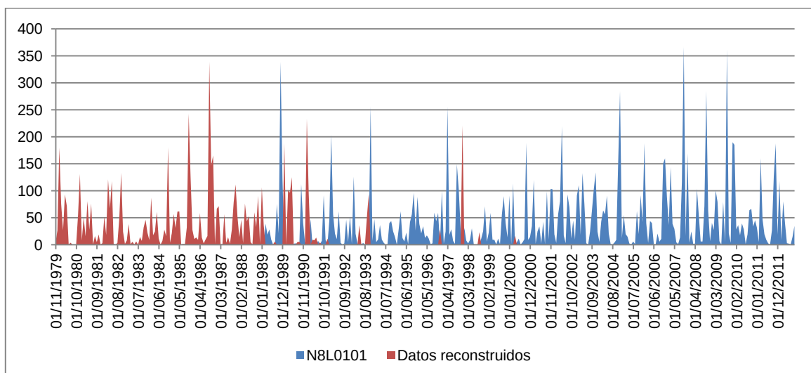
Figura 42. Serie de precipitación mensual completada (mm) del pluviómetro Aforo en Sistema Marina Baixa (N8L0101).
