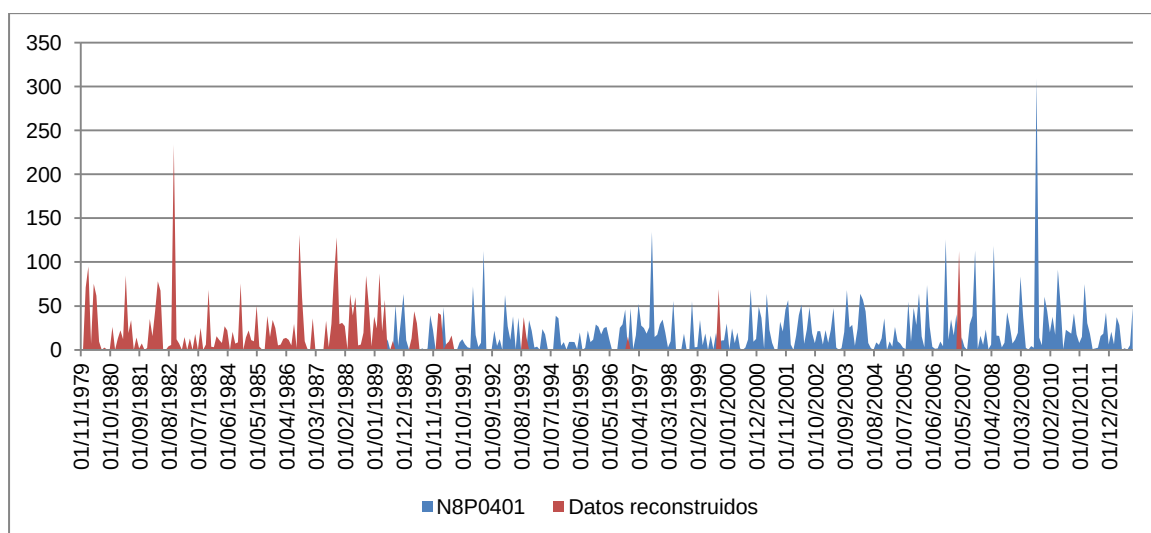
Figura 58. Serie de precipitación mensual completada (mm) del pluviómetro Agost (N8P0401).
