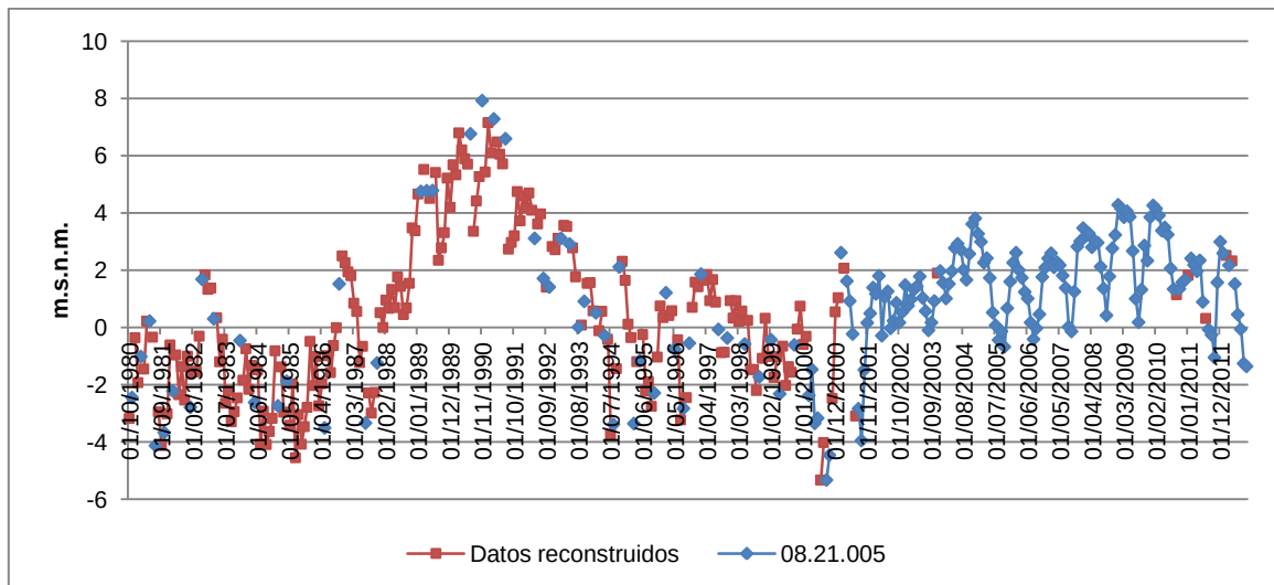
Figura 82. Serie de piezometría mensual completada del piezómetro de Sagunto (08.21.005).
