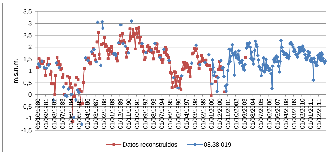
Figura 90. Serie de piezometría mensual completada del piezómetro de Gandia (08.38.019).
