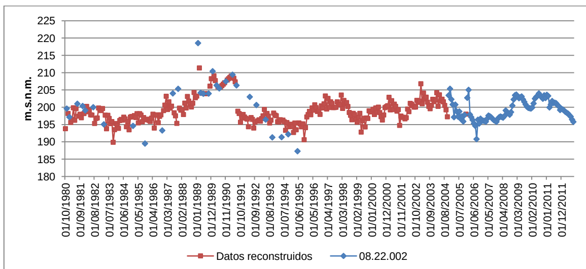
Figura 83. Serie de piezometría mensual completada del piezómetro de Bugarra (08.22.002).
