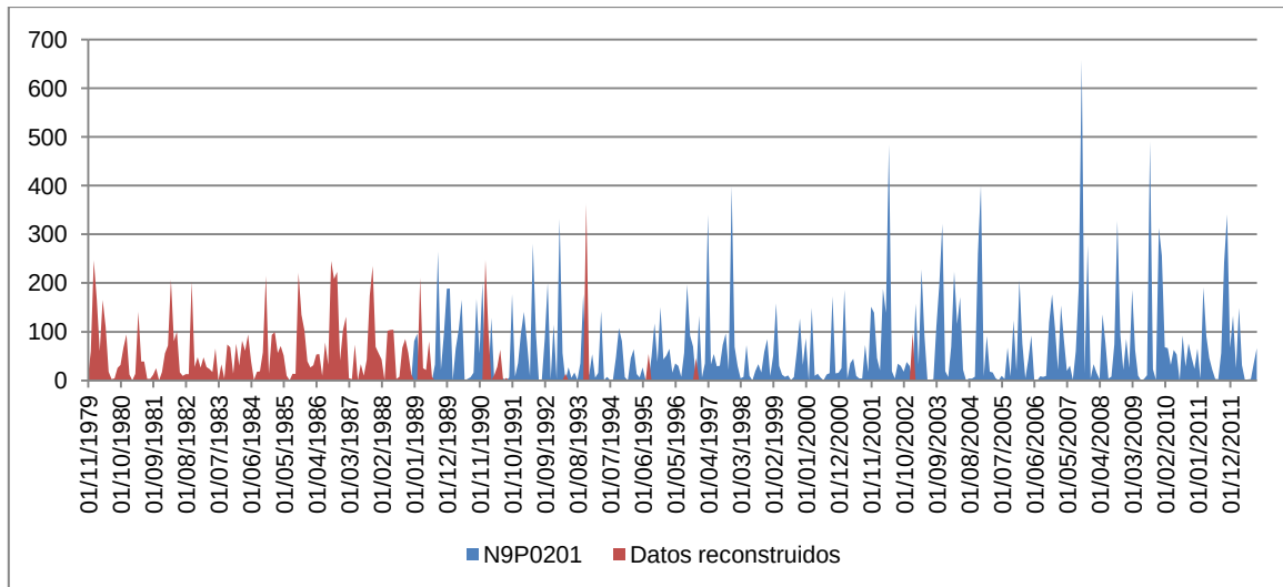
Figura 40. Serie de precipitación mensual completada (mm) del pluviómetro Alcalalí (N9P0201).
