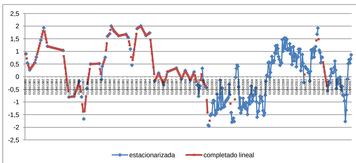
Figura 69. Serie estacionarizada y completada mediante interpolación lineal del piezómetro de Montesa (08.28.007).
