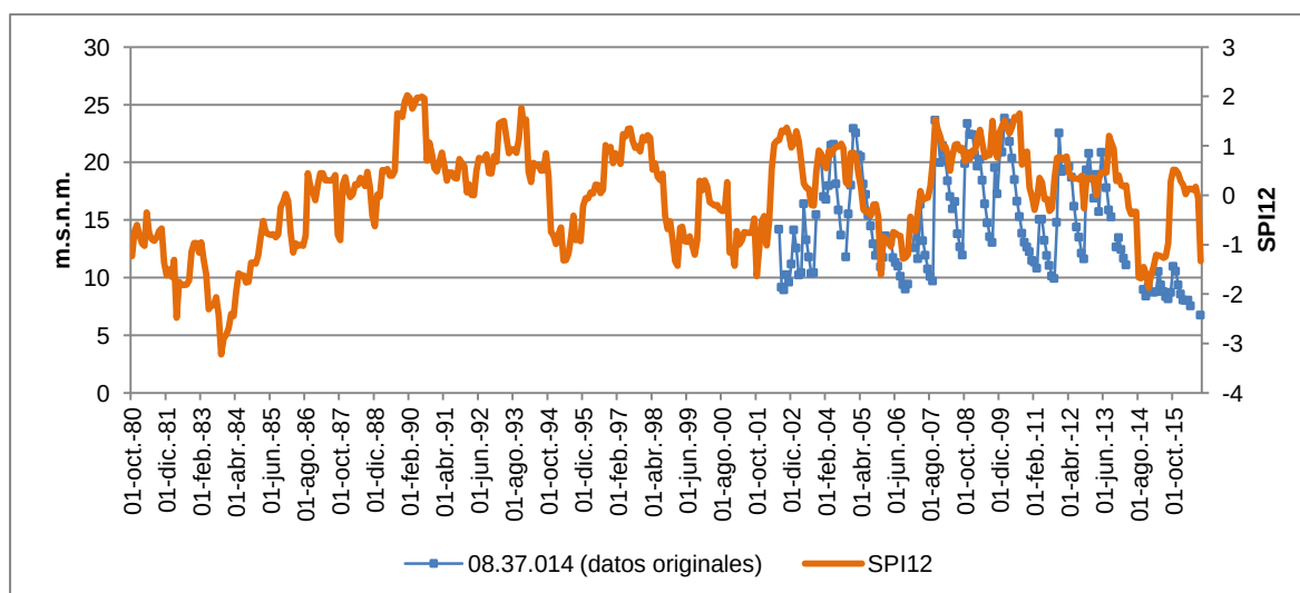
Figura 72. Serie de piezometría mensual original del piezómetro de Pego (08.37.014) y datos del SPI12.
