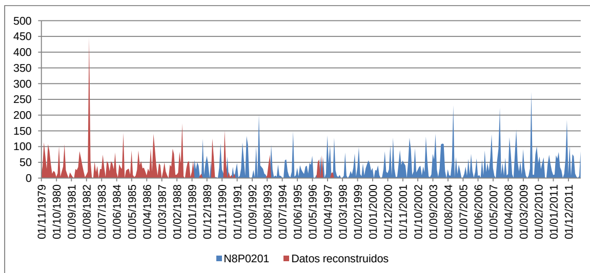
Figura 44. Serie de precipitación mensual completada (mm) del pluviómetro Benejama (N8P0201).
