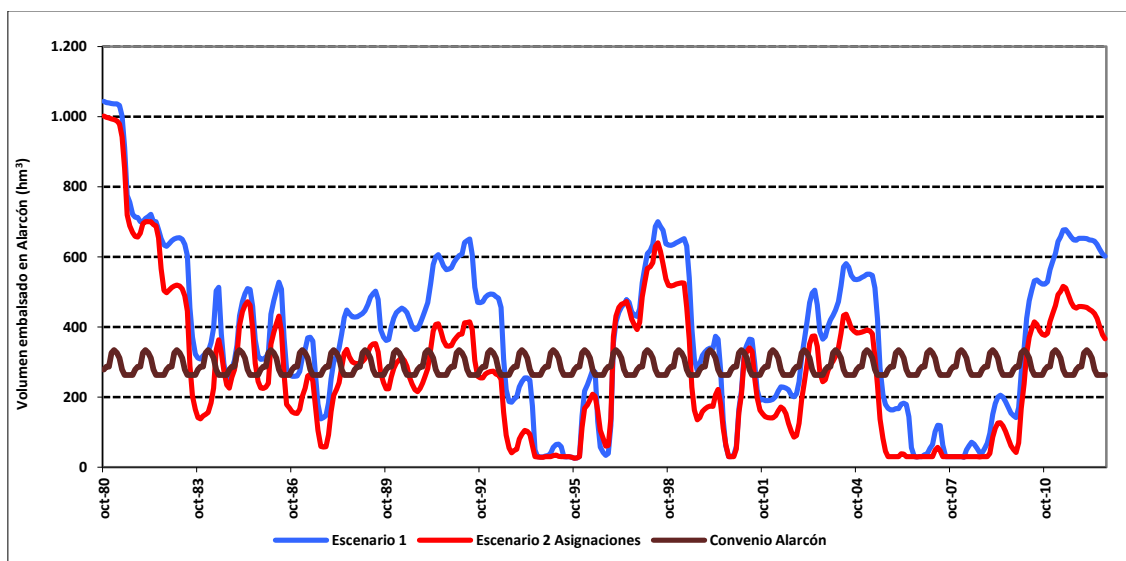
Figura 128. Volumen embalsado en Alarcón en el escenario 2 asignaciones respecto al escenario 1.
