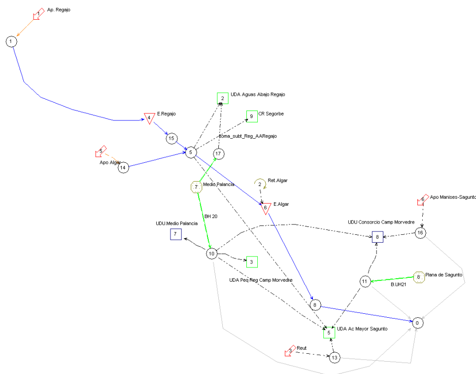
Figura 66. Esquema del modelo de simulación del sistema de explotación Palancia-Los Valles.
