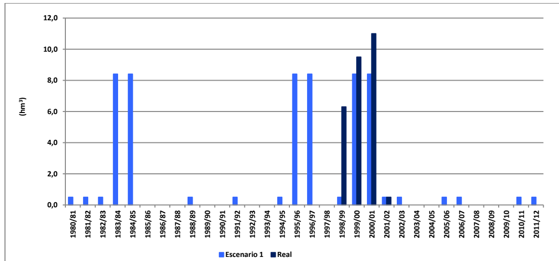
Figura 204. Volumen transferido mediante conducción Rabasa-Fenollar-Amadorio: escenario 1.
