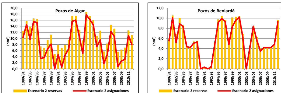
Figura 213. Series anuales de bombeos en los pozos de Algar y de Beniardá en el escenario 2 reservas respecto al escenario 2 asignaciones.
