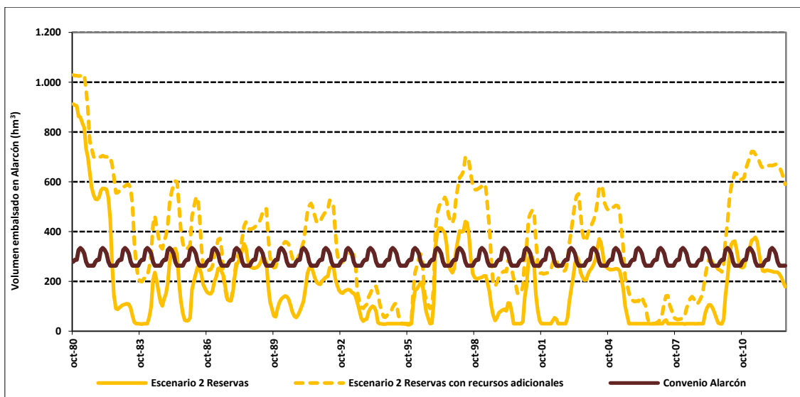
Figura 136. Volumen embalsado en Alarcón en el escenario 2 reservas con y sin recursos adicionales.
