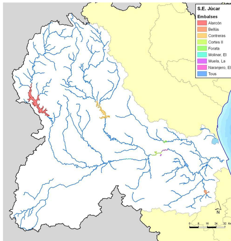
Figura 106. Embalses del sistema de explotación Júcar.
