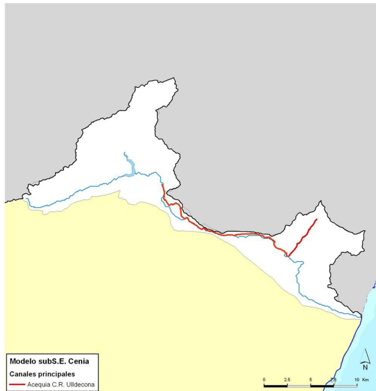
Figura 12. Canales considerados en el modelo de simulación del subsistema de explotación Cenia.
