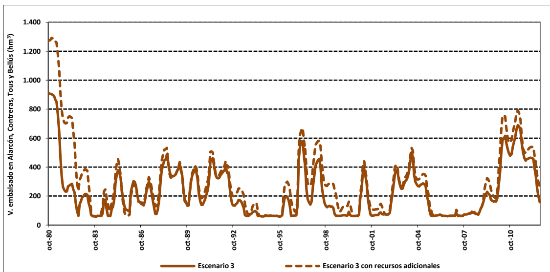
Figura 143. Volumen embalsado en Alarcón, Contreras, Tous y Bellús en el escenario 4 con y sin recursos adicionales.
