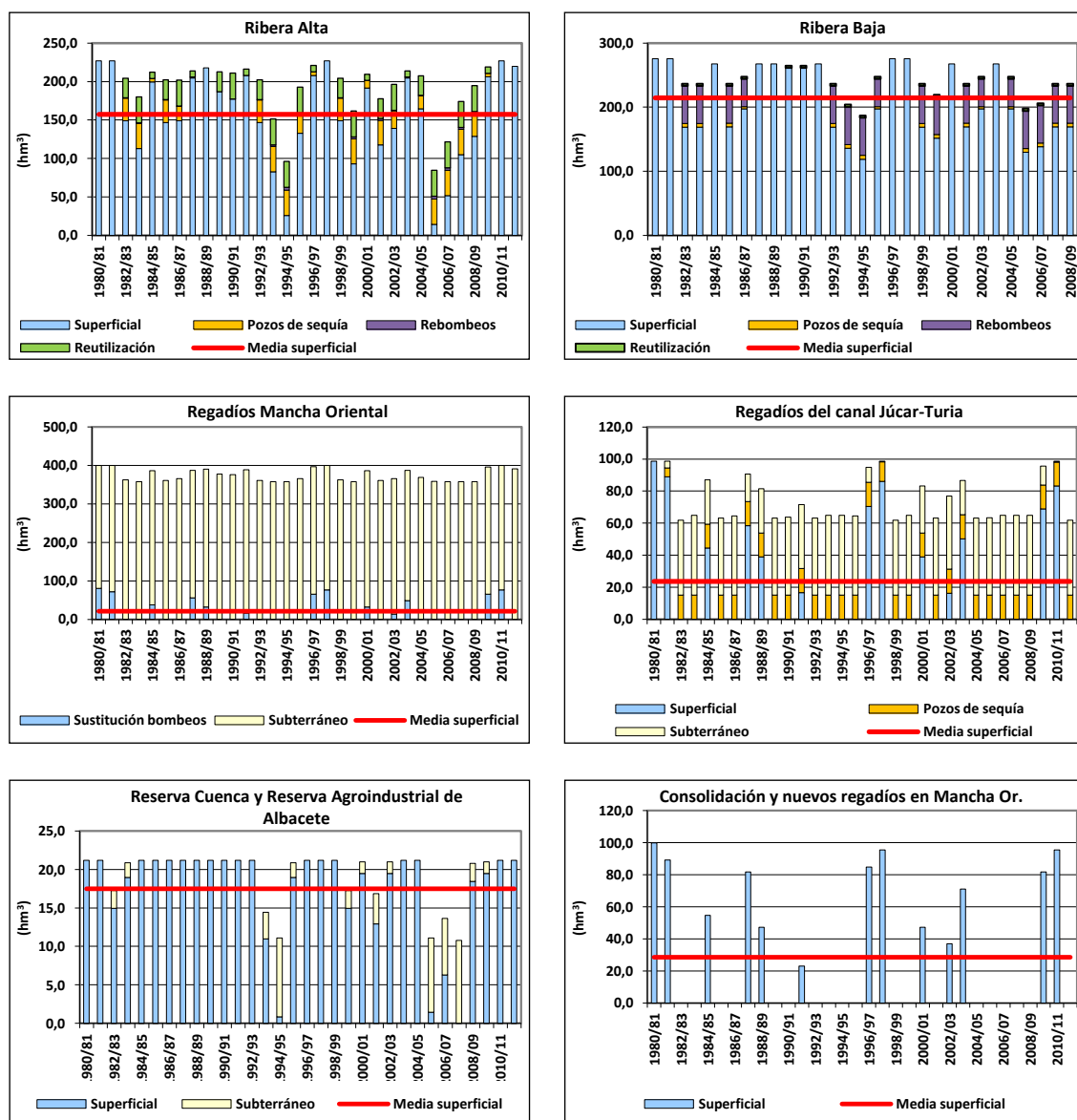
Figura 133. Series anuales de suministro a las principales demandas del sistema de explotación Júcar por origen de los recursos: escenario 2 reservas.
