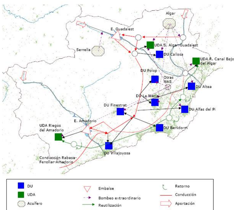
Figura 189. Esquema conceptual del sistema de explotación Marina Baja.
