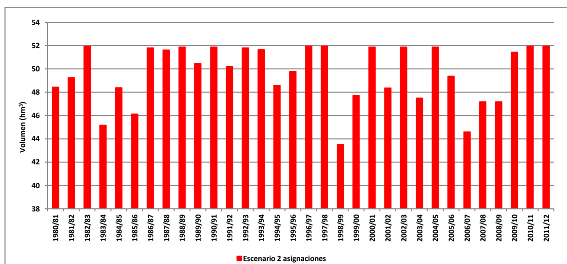
Figura 130. Volumen transferido por la conducción Júcar-Vinalopó con capacidad de 2,6 \text{ m}^3/\text{s} y régimen de no riego: escenario 2 asignaciones.
