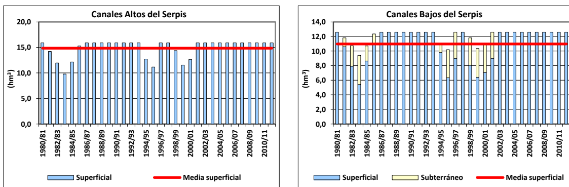
Figura 165. Series anuales de suministro a las principales demandas del sistema de explotación Serpis por origen de los recursos: escenario 1.
