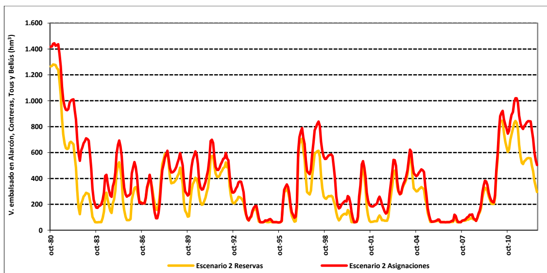
Figura 131. Volumen embalsado en Alarcón, Contreras, Tous y Bellús en el escenario 2 reservas respecto al escenario 2 asignaciones.
