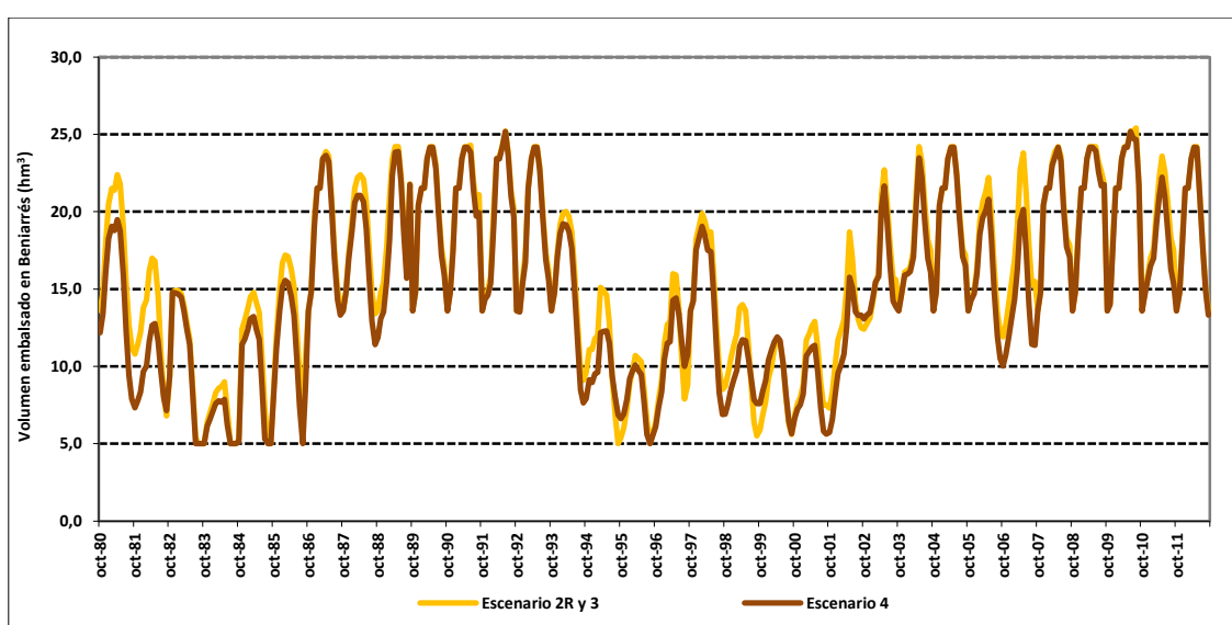
Figura 170. Volumen embalsado en Beniarrés en el escenario 4 respecto al escenario 3.
