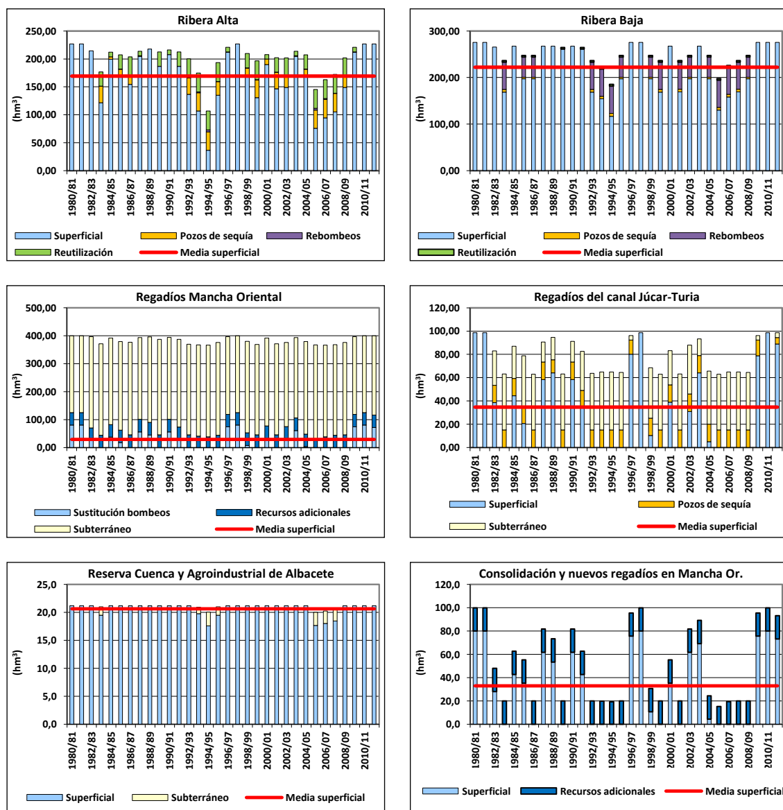
Figura 145. Series anuales de suministro a las principales demandas del sistema de explotación Júcar por origen de los recursos: escenario 4 con recursos adicionales.
