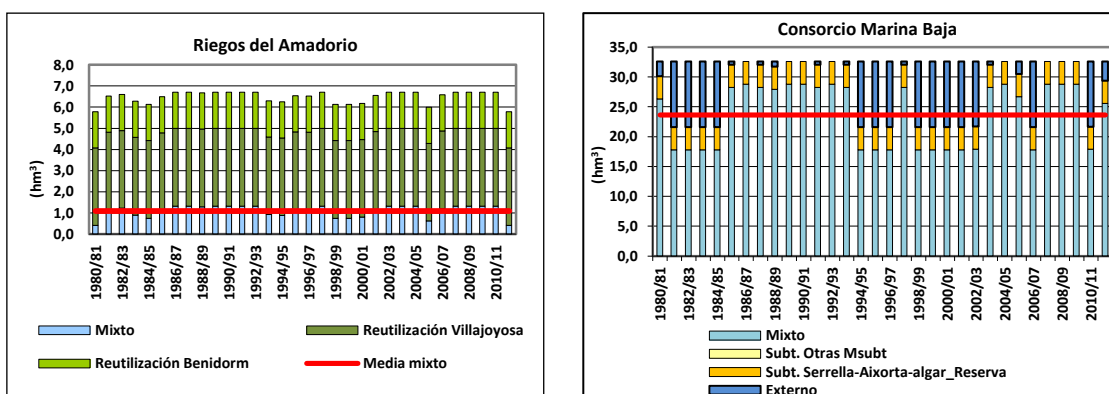
Figura 212. Series anuales de suministro a las principales demandas del sistema de explotación Marina Baja por origen de los recursos: escenario 2 reservas.
