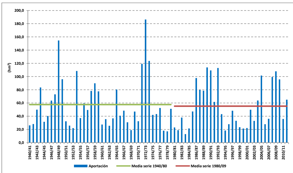
Figura 157. Aportación anual total en el modelo de simulación del sistema de explotación Serpis.
