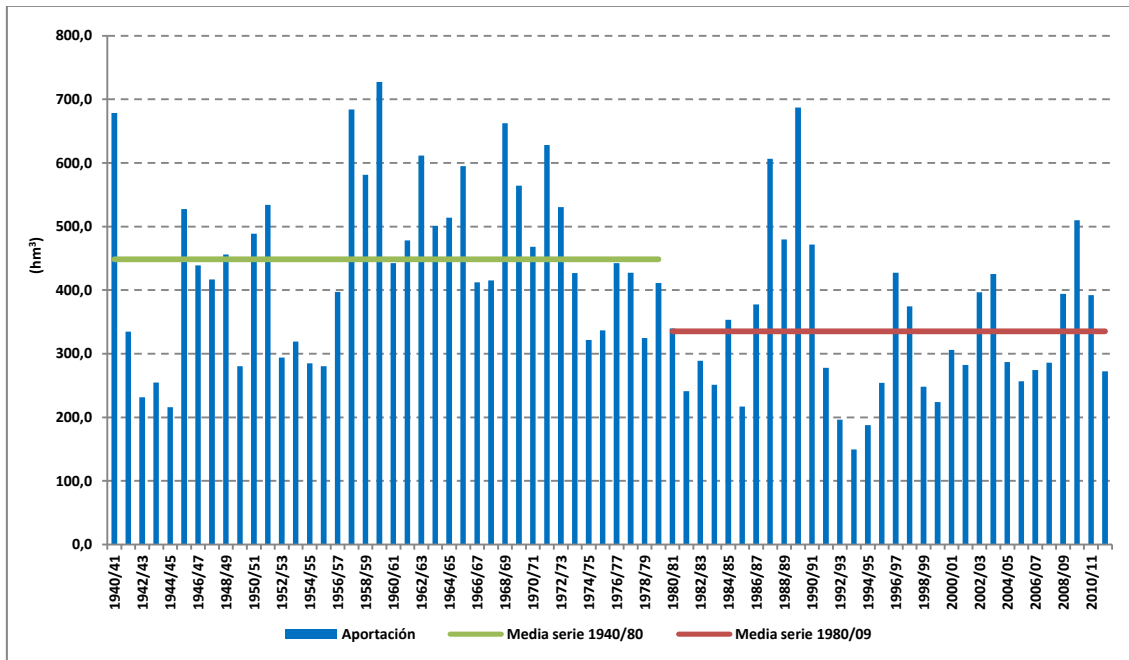
Figura 88. Aportación anual total en el modelo de simulación del sistema de explotación Turia.
