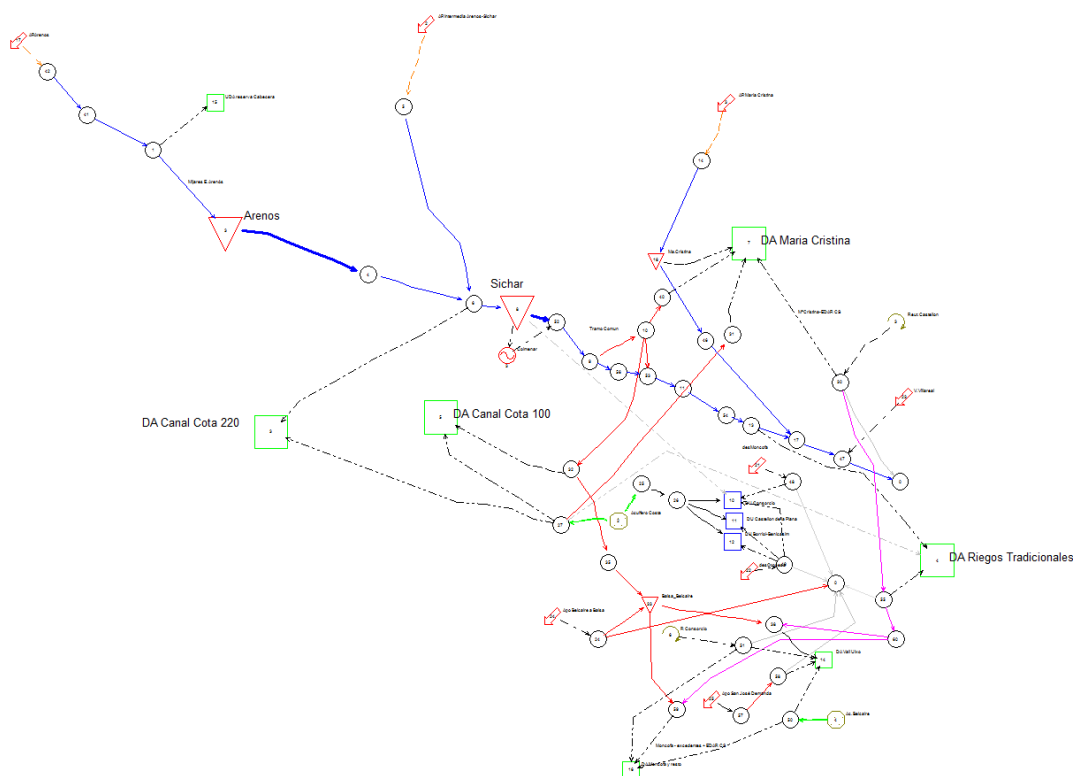
Figura 40. Esquema del modelo de simulación del sistema de explotación Mijares-Plana de Castellón: escenario 1.
