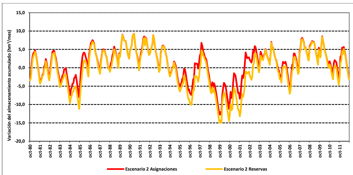
Figura 215. Variación del almacenamiento acumulado en el acuífero de Algar en escenario 2 reservas frente al escenario 2 asignaciones.
