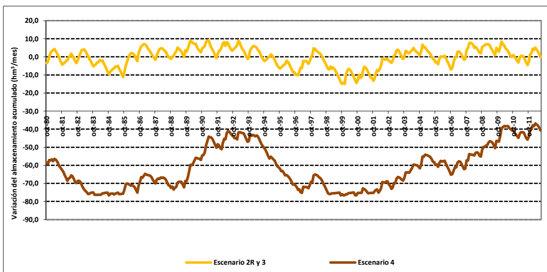
Figura 221. Variación del almacenamiento acumulado en el acuífero de Algar en escenario 4 frente al escenario 2R y 3.
