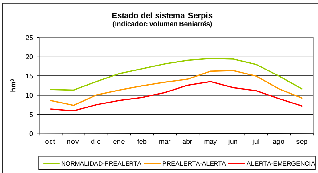
Figura 163. Curvas de estado para el sistema de explotación Serpis.
