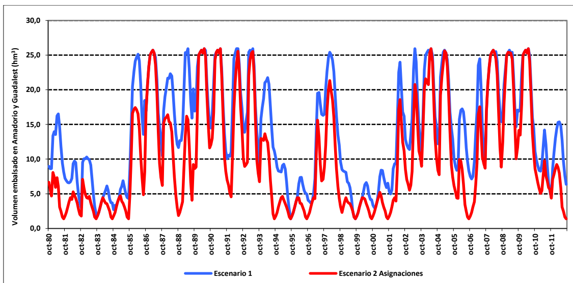
Figura 205. Volumen embalsado en Amadorio y Guadalest en el escenario 2 asignaciones respecto al escenario 1.
