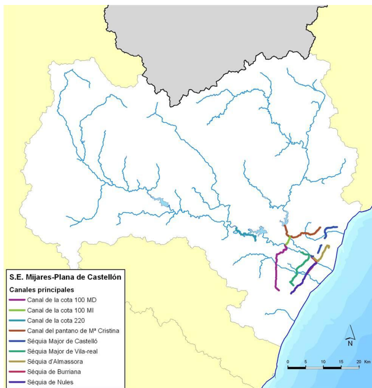
Figura 28. Conducciones de transporte principales del sistema de explotación Mijares-Plana de Castellón.
