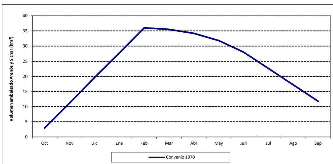
Figura 47. Curva empleada en la gestión del río Mijares: escenario 2 reservas.
