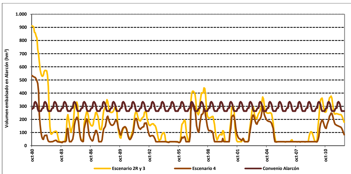
Figura 140. Volumen embalsado en Alarcón en el escenario 4 respecto al escenario 2R y 3.
