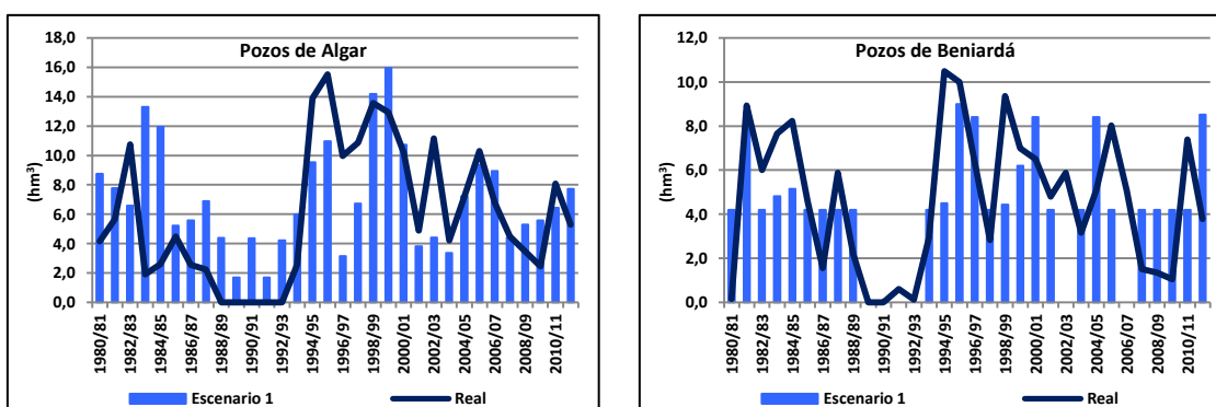
Figura 203. Series anuales de bombeos en los pozos de Algar y de Beniardá: escenario 1.
