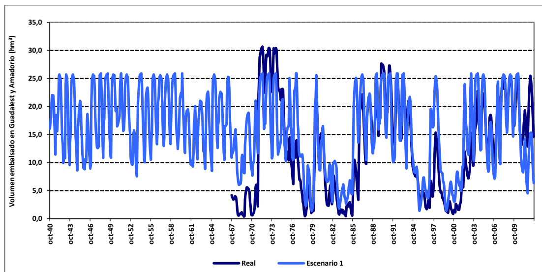
Figura 201. Calibración modelo del sistema de explotación Marina Baja.
