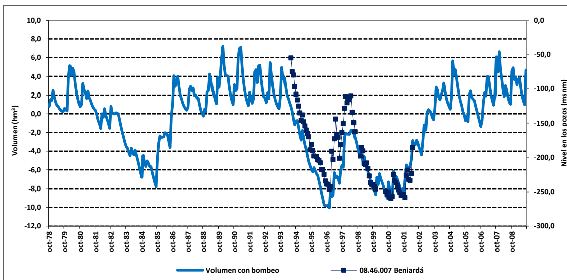
Figura 194. Volumen almacenado en el acuífero de Serrella, modelado como acuífero con manantial.
