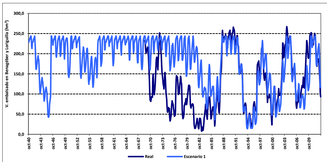
Figura 94. Calibración modelo del sistema de explotación Turia.
