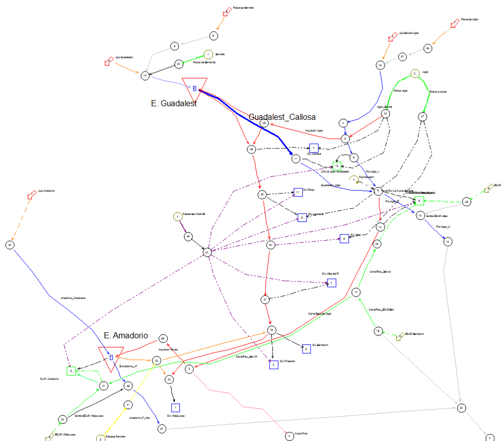
Figura 199. Esquema del modelo de simulación del sistema de explotación Marina Baja.
