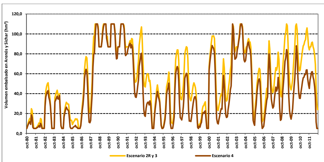
Figura 49. Volumen embalsado en Arenós y Sichar en el escenario 4 respecto al escenario 2R y 3.
