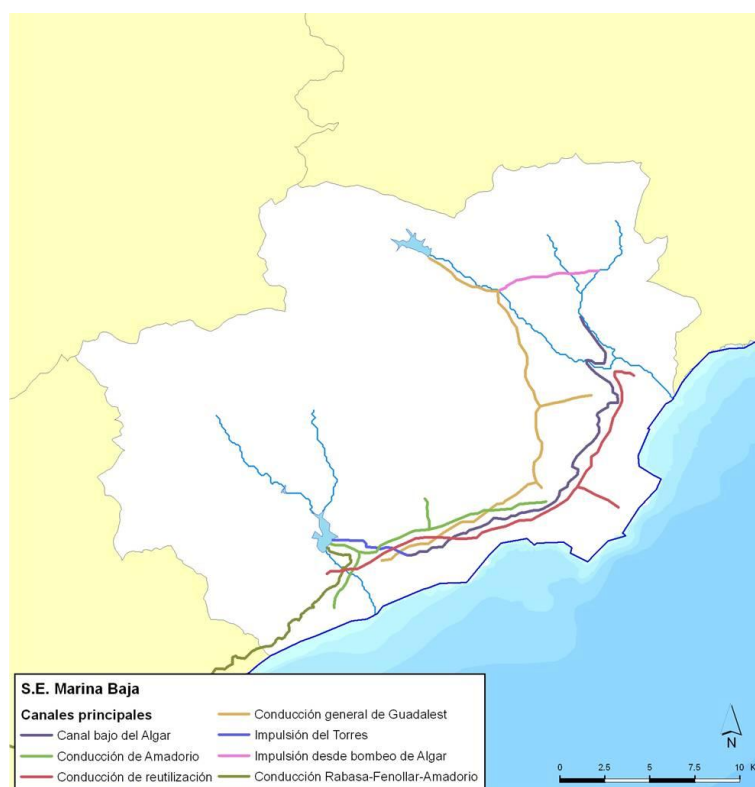
Figura 182. Conducciones de transporte principales del sistema de explotación Marina Baja.
