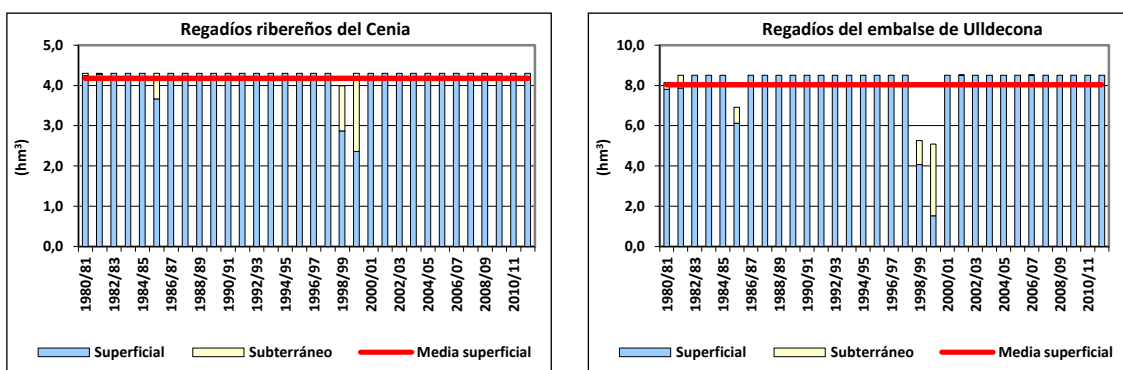
Figura 22. Series anuales de suministro a las principales demandas del subsistema de explotación Cenia por origen de los recursos: escenario 2 asignaciones.
