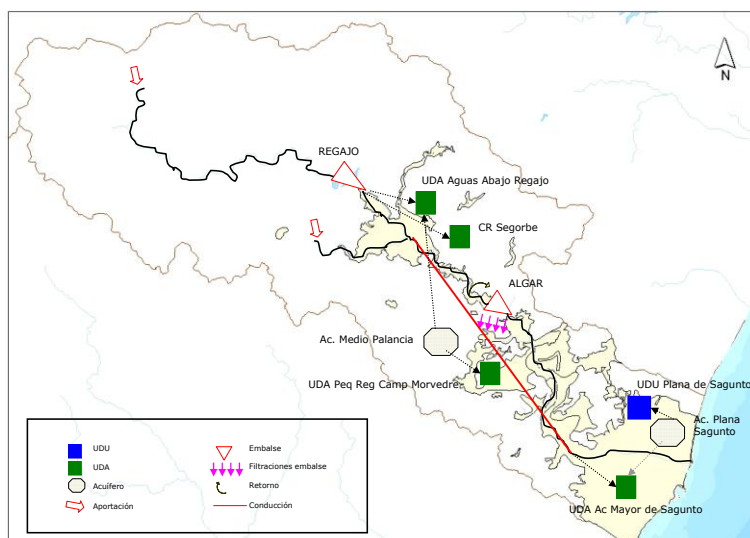
Figura 59. Esquema conceptual del sistema de explotación Palancia - Los Valles.
