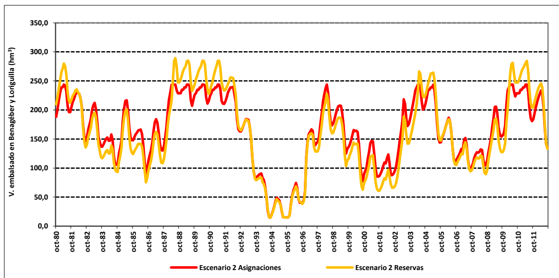
Figura 98. Volumen embalsado en Benagéber y Loriguilla en el escenario 2 reservas respecto al escenario 2 asignaciones.
