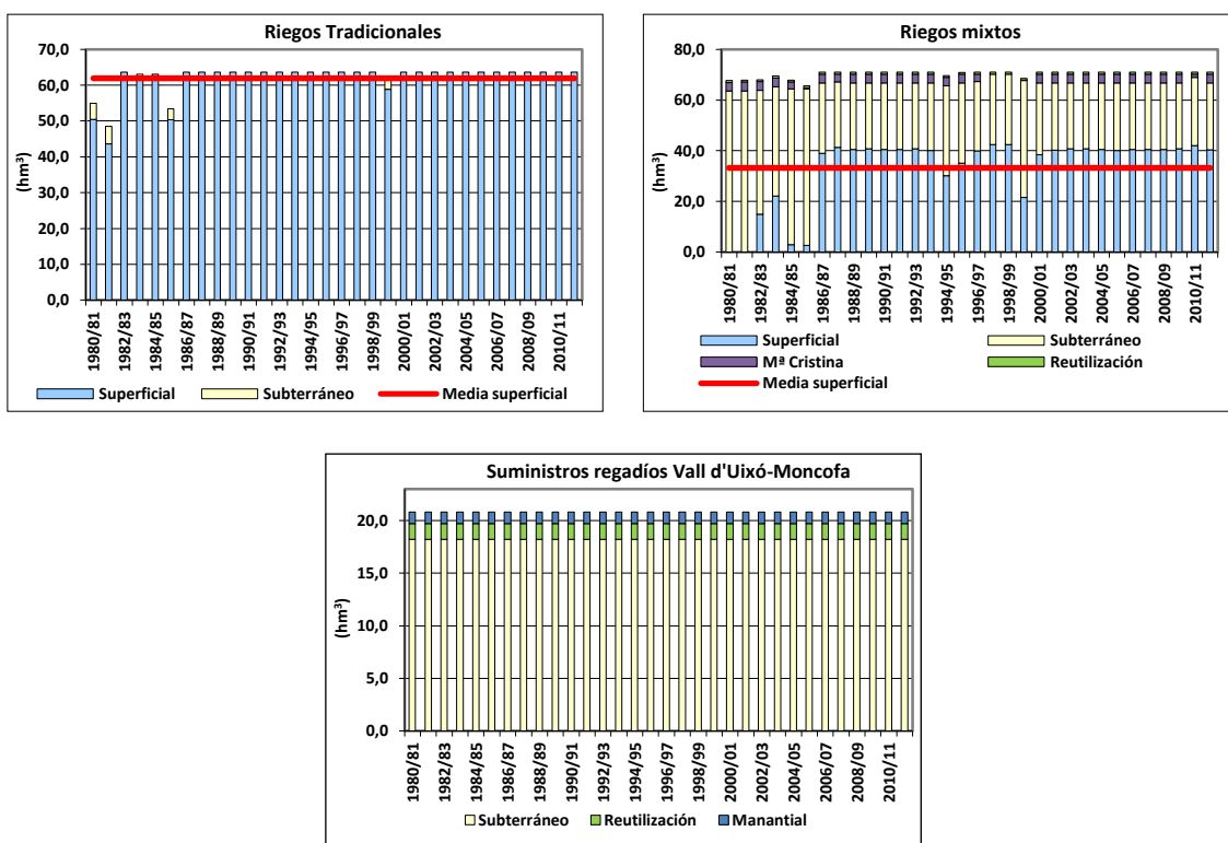
Figura 43. Series anuales de suministro a las principales demandas del sistema de explotación Mijares-Plana de Castellón por origen de los recursos: escenario 1.
