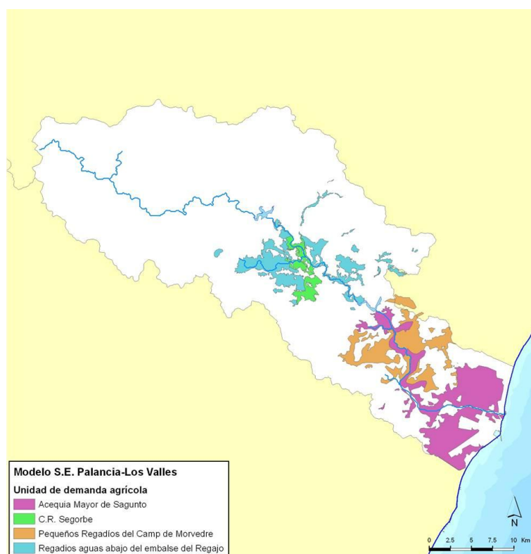
Figura 65. UDA consideradas en el modelo de simulación del sistema de explotación Palancia-Los Valles.
