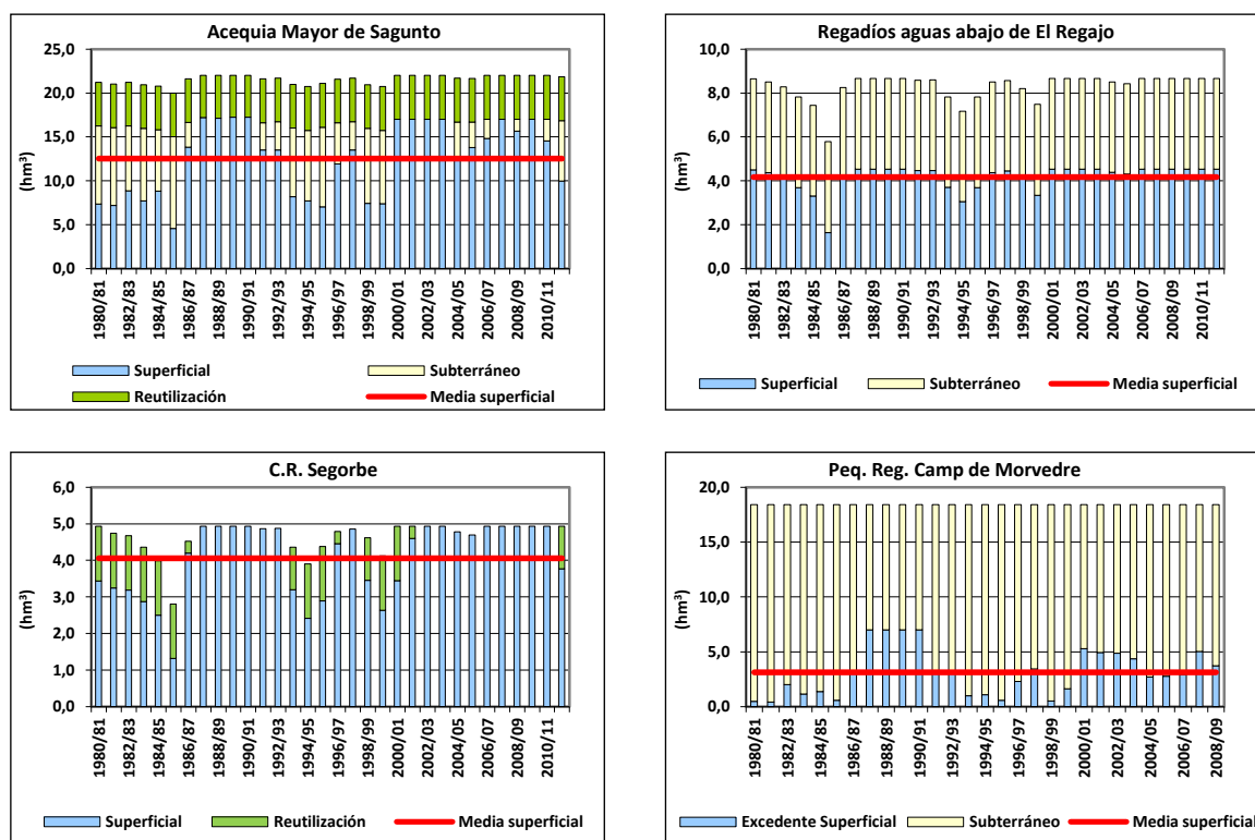
Figura 76. Series anuales de suministro a las principales demandas agrícolas del sistema de explotación Palancia-Los Valles por origen de los recursos: escenario 4.
