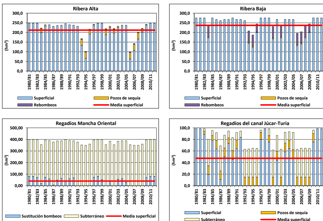
Figura 129. Series anuales de suministro a las principales demandas del sistema de explotación Júcar por origen de los recursos: escenario 2 asignaciones.
