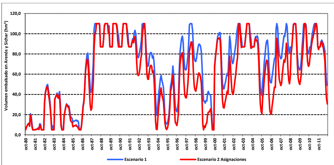
Figura 44. Volumen embalsado en Arenós y Schar en el escenario 2 asignaciones respecto al escenario 1.
