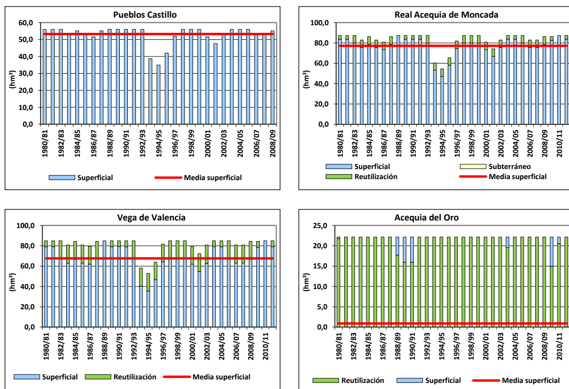
Figura 95. Series anuales de suministro a las principales demandas del sistema de explotación Turia por origen de los recursos: escenario 1.
