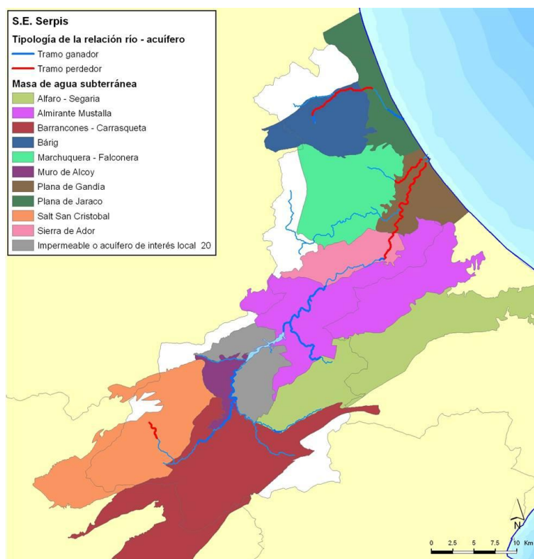
Figura 150. Tipología de la relación río-acuífero en el sistema de explotación Serpis.
