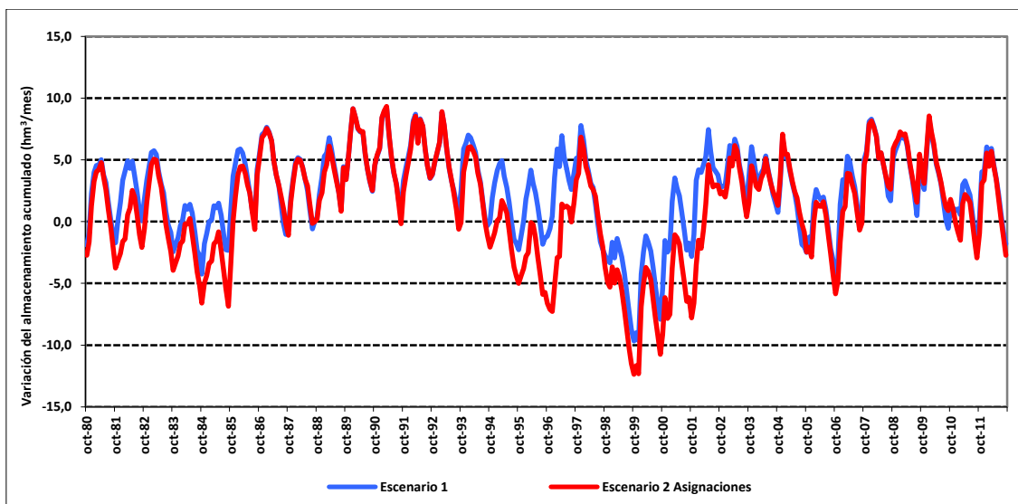
Figura 209. Variación del almacenamiento acumulado en el acuífero de Algar en escenario 2 asignaciones frente al escenario 1.
