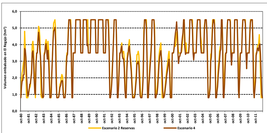
Figura 75. Volumen embalsado en El Regajo en el escenario 4 respecto al escenario 2 reservas.
