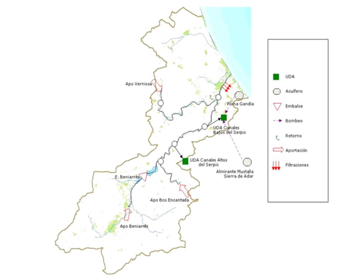
Figura 155. Esquema conceptual del sistema de explotación Serpis.
