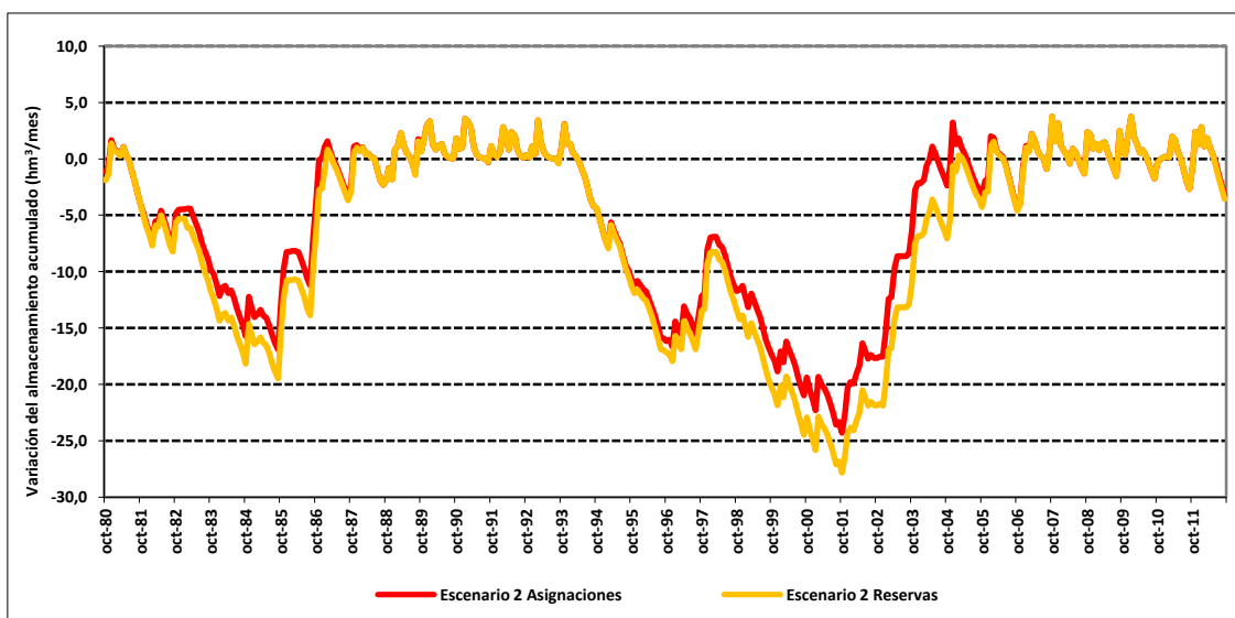
Figura 214. Variación del almacenamiento acumulado en el acuífero de Serrella en escenario 2 reservas frente al escenario 2 asignaciones.
