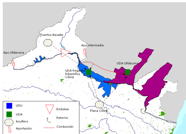
Figura 11. Esquema conceptual del subsistema explotación Cenia.
