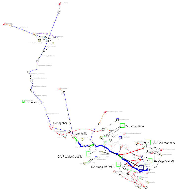
Figura 93. Esquema del modelo de simulación del sistema de explotación Turia: escenario 1.
