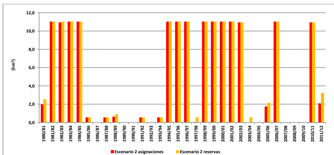
Figura 216. Volumen transferido mediante conducción Rabasa-Fenollar-Amadorio en el escenario 2 reservas frente al escenario 2 asignaciones.
