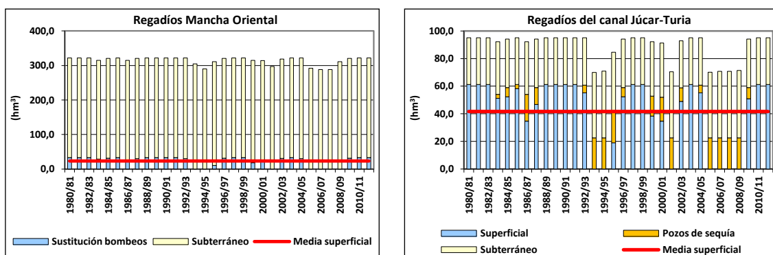
Figura 126. Series anuales de suministro a las principales demandas del sistema de explotación Júcar por origen de los recursos: escenario 1.
