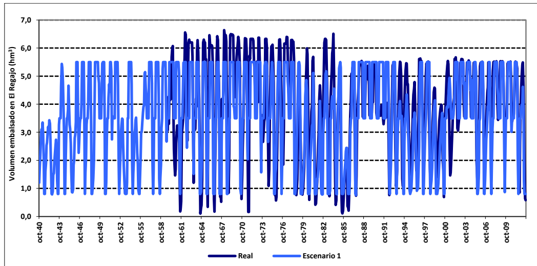
Figura 68. Calibración modelo del sistema de explotación Palancia-Los Valles.
