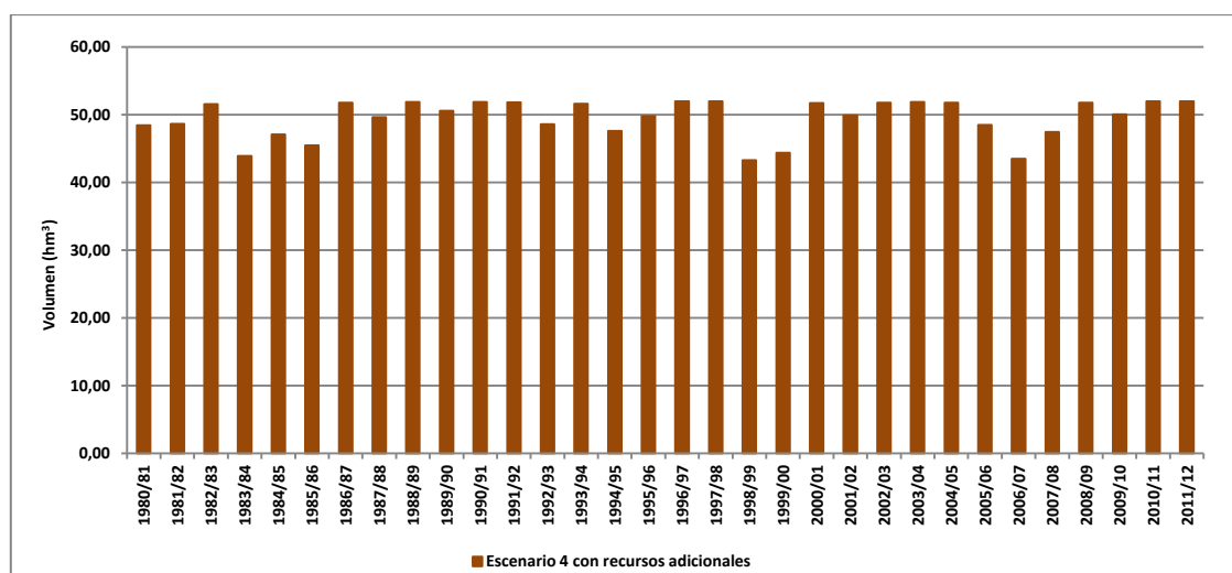
Figura 146. Volumen transferido por la conducción Júcar-Vinalopó con capacidad de 2,6 \text{ m}^3/\text{s} y régimen de no riego: escenario 4 con recursos adicionales.
