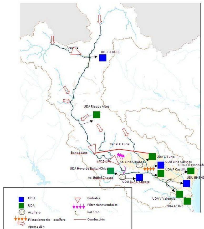
Figura 86. Esquema conceptual del sistema de explotación Turia.
