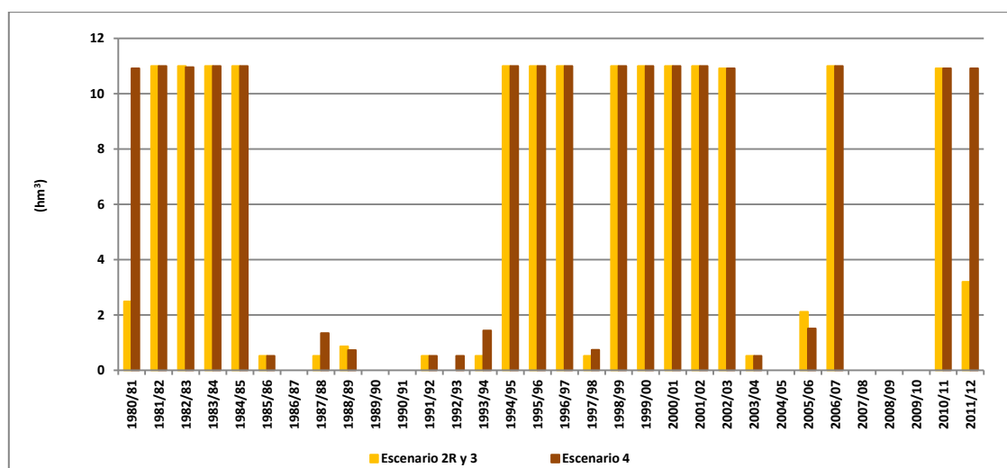
Figura 222. Volumen transferido mediante conducción Rabasa-Fenollar-Amadorio en el escenario 4 frente al escenario 2R y 3.
