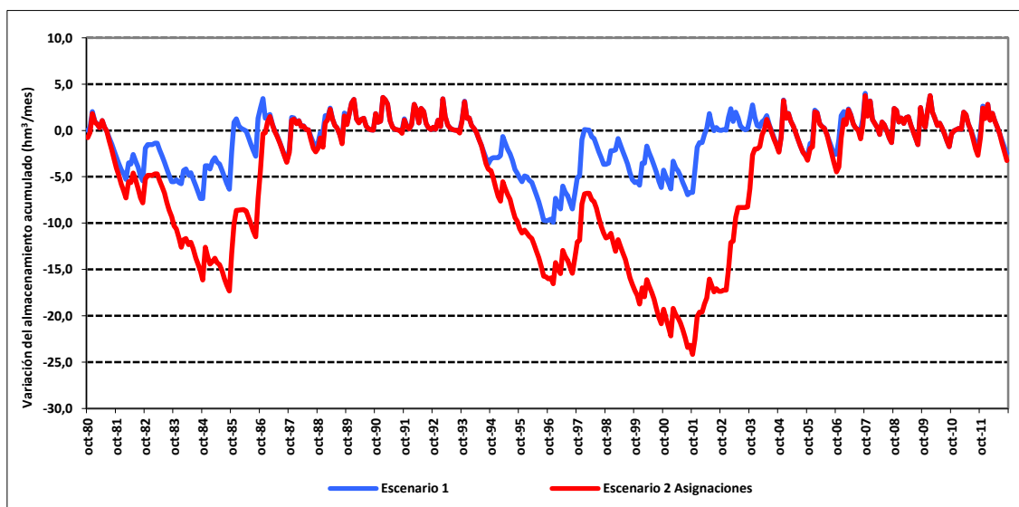
Figura 208. Variación del almacenamiento acumulado en el acuífero de Serrella en escenario 2 asignaciones frente al escenario 1.
