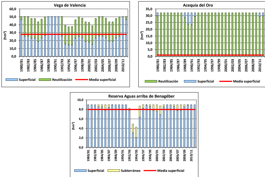
Figura 103. Series anuales de suministro a las principales demandas del sistema de explotación Turia por origen de los recursos: escenario 4.
