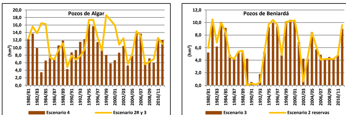
Figura 219. Series anuales de bombeos en los pozos de Algar y de Beniardá en el escenario 4 respecto al escenario 2 reservas y 3.
