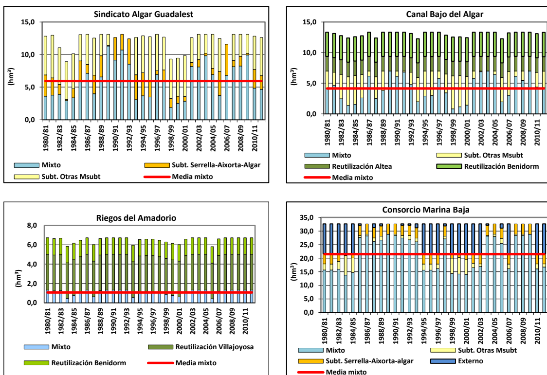
Figura 218. Series anuales de suministro a las principales demandas del sistema de explotación Marina Baja por origen de los recursos: escenario 4.
