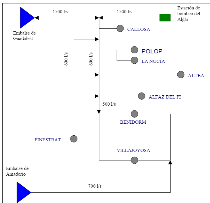
Figura 190. Esquema de la red de abastecimiento de la Marina Baja.
