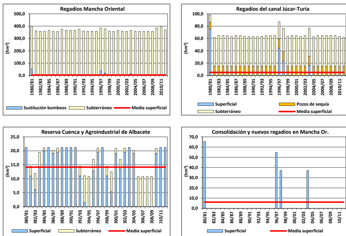
Figura 141. Series anuales de suministro a las principales demandas del sistema de explotación Júcar por origen de los recursos: escenario 4.
