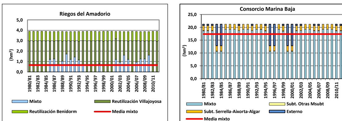
Figura 202. Series anuales de suministro a las principales demandas del sistema de explotación Marina Baja por origen de los recursos: escenario 1.
