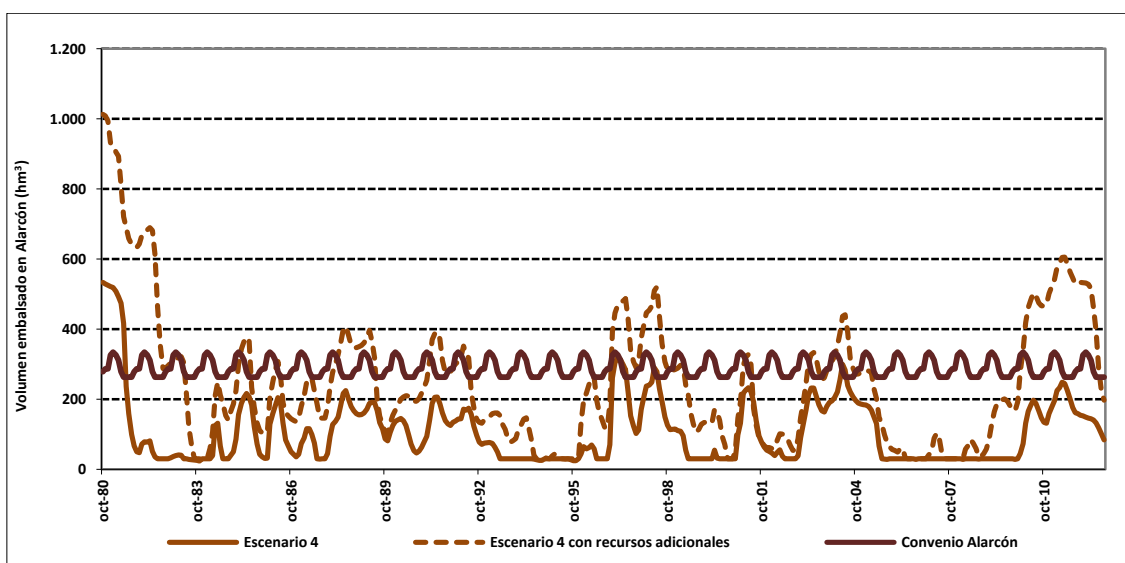
Figura 144. Volumen embalsado en Alarcón en el escenario 4 con y sin recursos adicionales.
