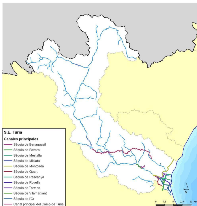
Figura 80. Conducciones de transporte principales del sistema de explotación Turia.
