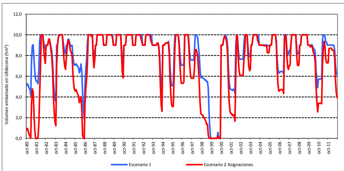
Figura 21. Volumen embalsado en Ulldecona en el escenario 2 asignaciones respecto al escenario 1.
