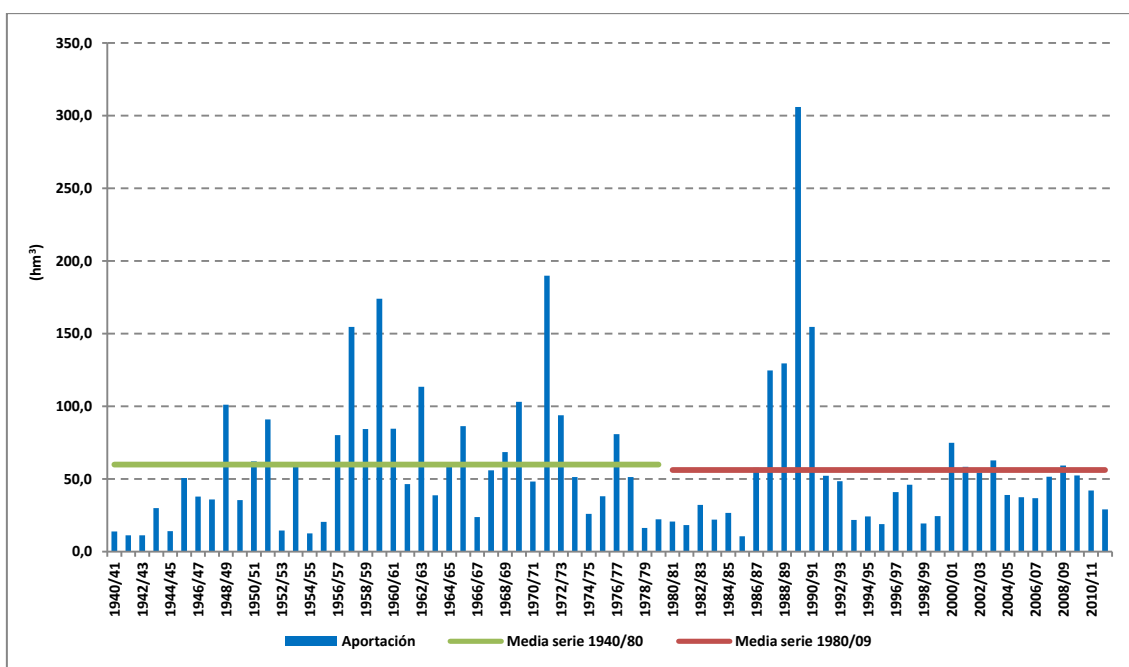
Figura 61. Aportación anual total en el modelo de simulación del sistema de explotación Palencia-Los Valles.
