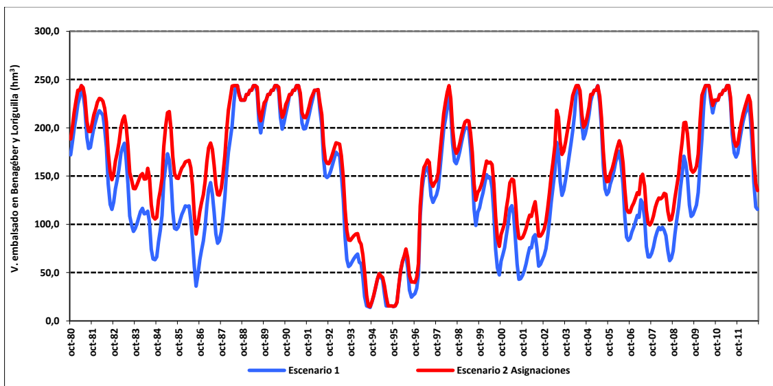
Figura 96. Volumen embalsado en Benagéber y Loriguilla en el escenario 2 asignaciones respecto al escenario 1.
