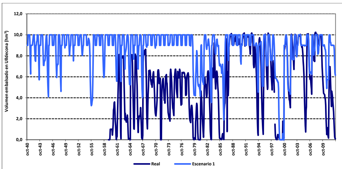
Figura 19. Calibración modelo de simulación del subsistema de explotación Cenia.
