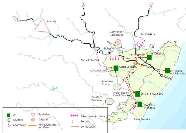
Figura 34. Esquema conceptual del sistema de explotación Mijares-Plana de Castellón
