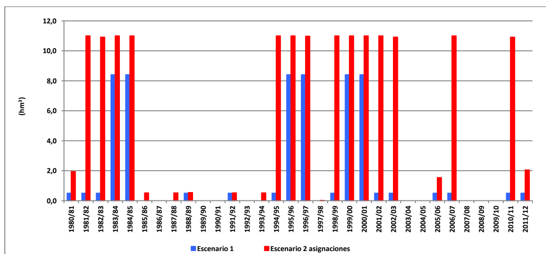
Figura 210. Volumen transferido mediante conducción Rabasa-Fenollar-Amadorio en el escenario 2 asignaciones frente al escenario 1.
