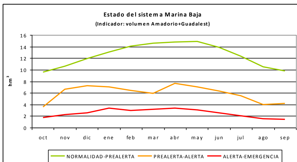
Figura 200. Curvas de estado para el sistema de explotación Marina Baja.
