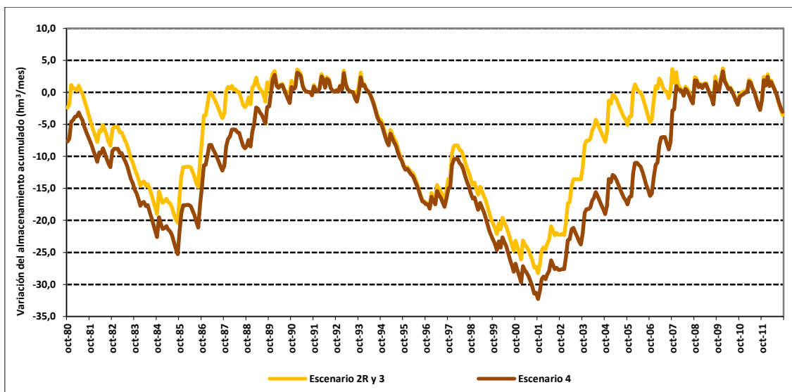
Figura 220. Variación del almacenamiento acumulado en el acuífero de Serrella en escenario 4 frente al escenario 2R y 3.
