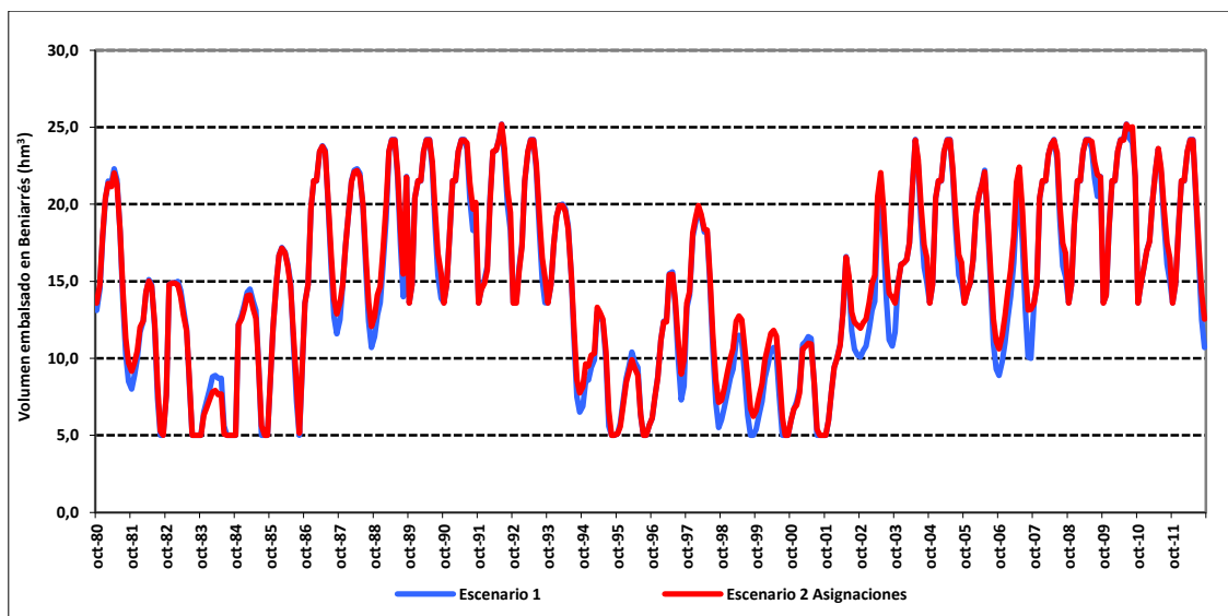
Figura 166. Volumen embalsado en Beniarrés en el escenario 2 asignaciones respecto al escenario 1.
