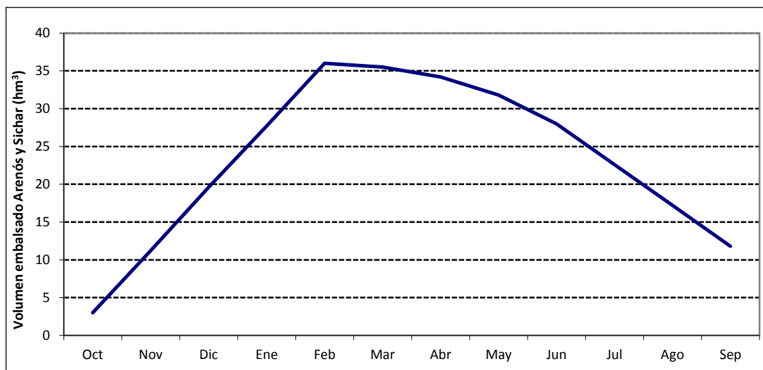
Figura 41. Curvas de restricciones para los riegos mixtos del Mijares.
