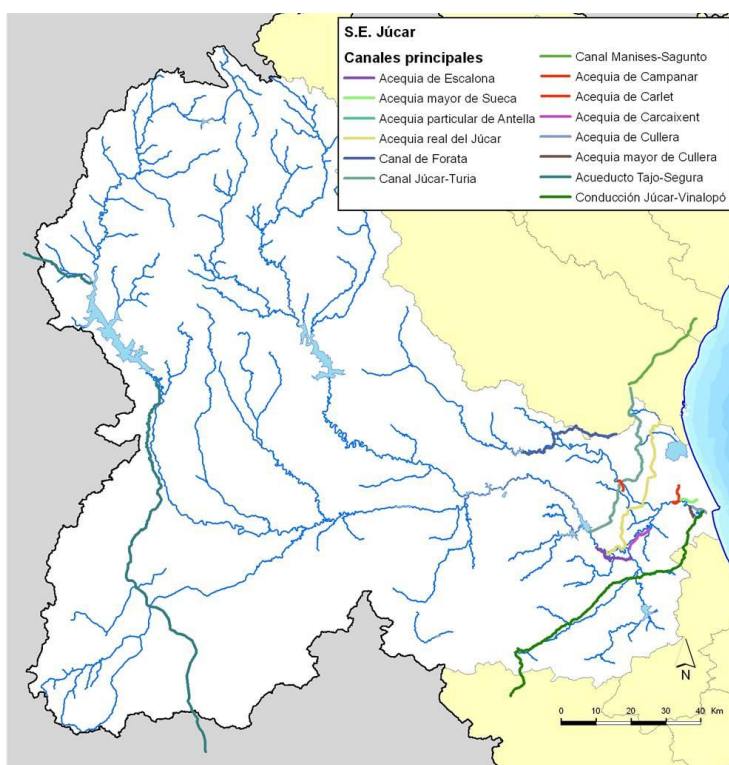
Figura 107. Conducciones de transporte principales del sistema de explotación Júcar.
