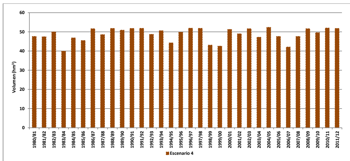
Figura 142. Volumen transferido por la conducción Júcar-Vinalopó con capacidad de 2,6 m 3 /s y régimen de no riego: escenario 4.
