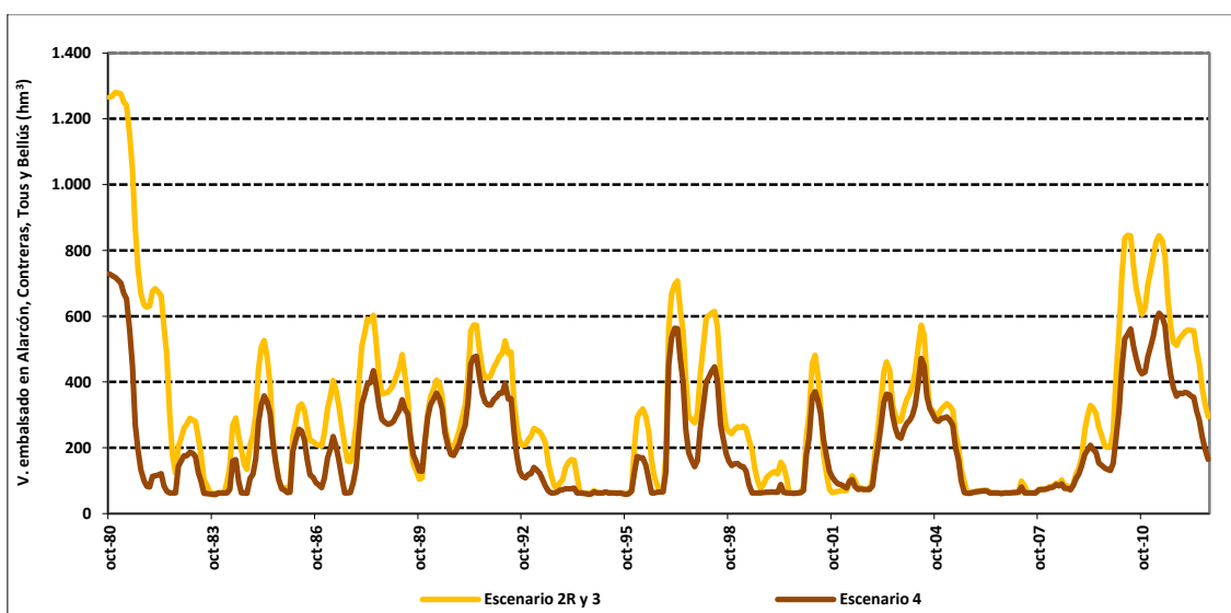
Figura 139. Volumen embalsado en Alarcón, Contreras, Tous y Bellús en el escenario 4 respecto al escenario 2R y 3.
