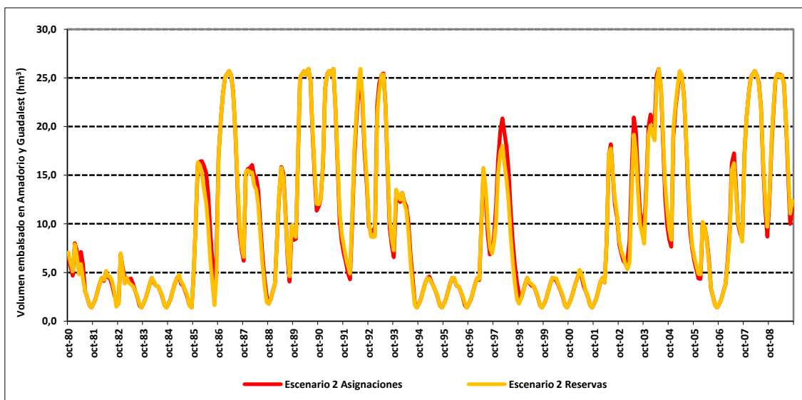
Figura 211. Volumen embalsado en Amadorio y Guadalest en el escenario 2 reservas respecto al escenario 2 asignaciones.
