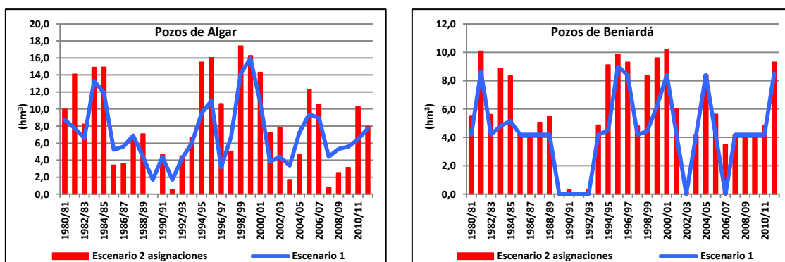
Figura 207. Series anuales de bombeos en los pozos de Algar y de Beniardá en el escenario 2 asignaciones respecto al escenario 1.
