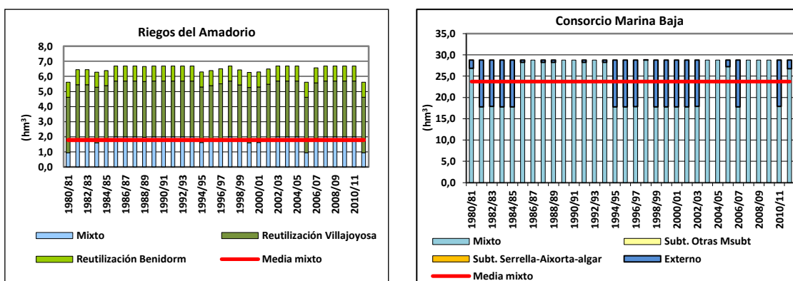
Figura 206. Series anuales de suministro a las principales demandas del sistema de explotación Marina Baja por origen de los recursos: escenario 2 asignaciones.
