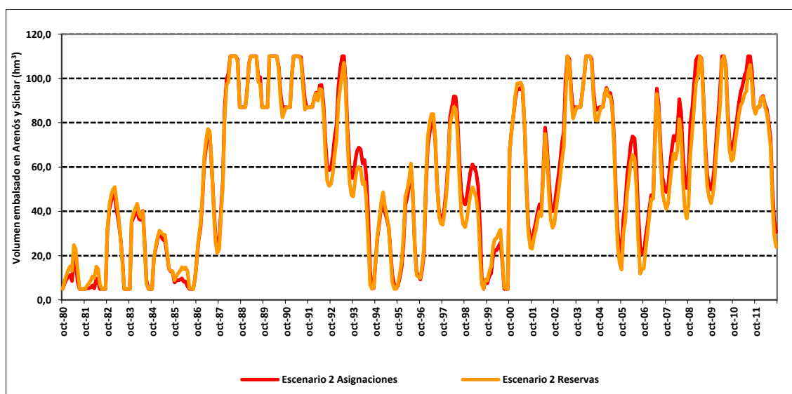
Figura 48. Volumen embalsado en Arenós y Schar en el escenario 2 reservas respecto al escenario 2 asignaciones.
