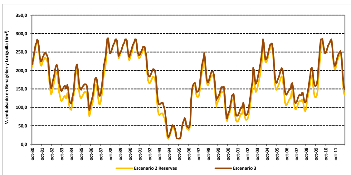
Figura 100. Volumen embalsado en Benagéber y Loriguilla en el escenario 3 respecto al escenario 2 reservas.
