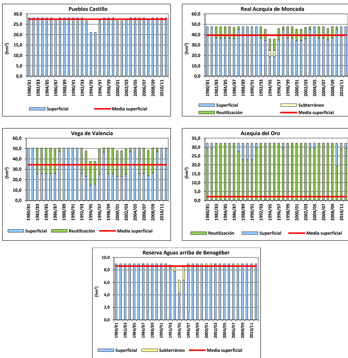
Figura 101. Series anuales de suministro a las principales demandas del sistema de explotación Turia por origen de los recursos: escenario 3.
