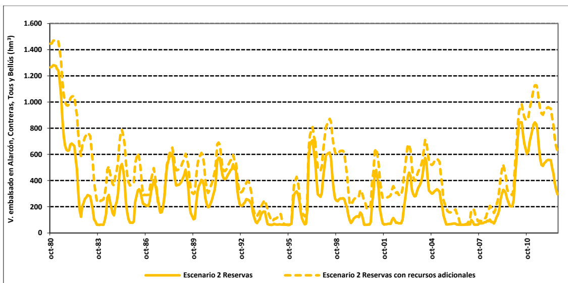
Figura 135. Volumen embalsado en Alarcón, Contreras, Tous y Bellús en el escenario 2 reservas con y sin recursos adicionales.
