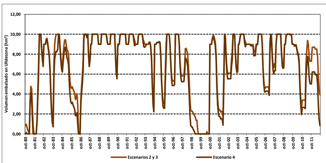
Figura 23. Volumen embalsado en Ulldecona en el escenario 4 respecto al escenario 2 y 3.
