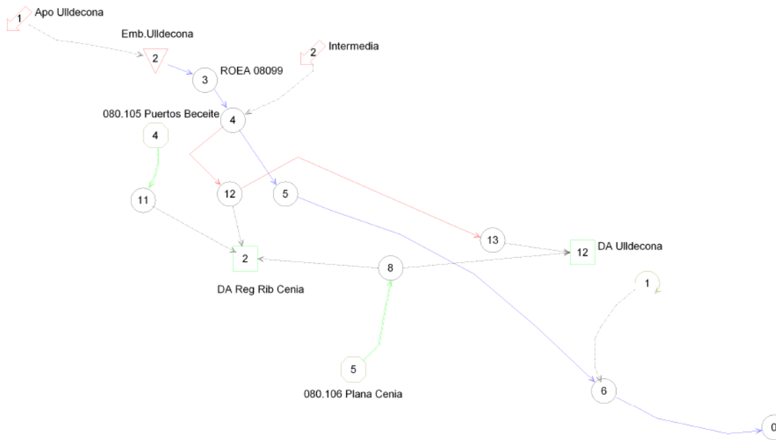
Figura 18. Esquema del modelo de simulación del subsistema de explotación Cenia: escenario 1.
