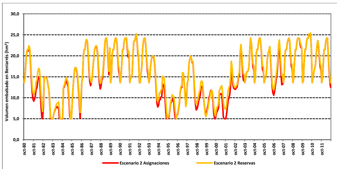
Figura 168. Volumen embalsado en Beniarrés en el escenario 2 reservas respecto al escenario 2 asignaciones.
