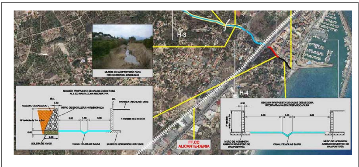
Planta del encauzamiento de la desembocadura (trazo negro)
