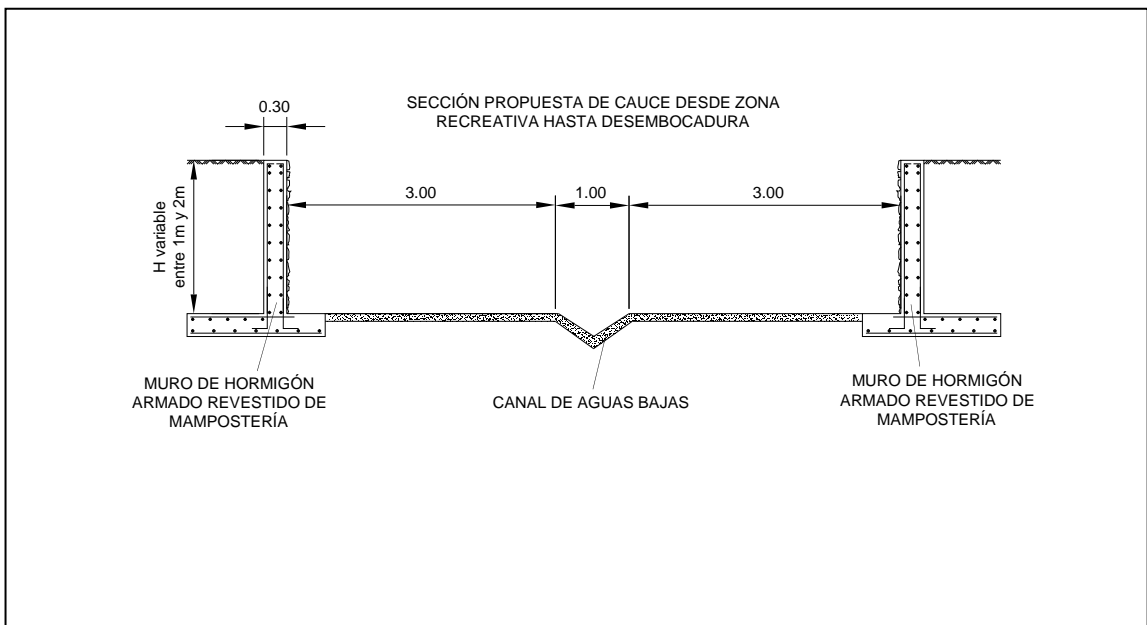
Sección tipo del encauzamiento en el tramo de desembocadura
