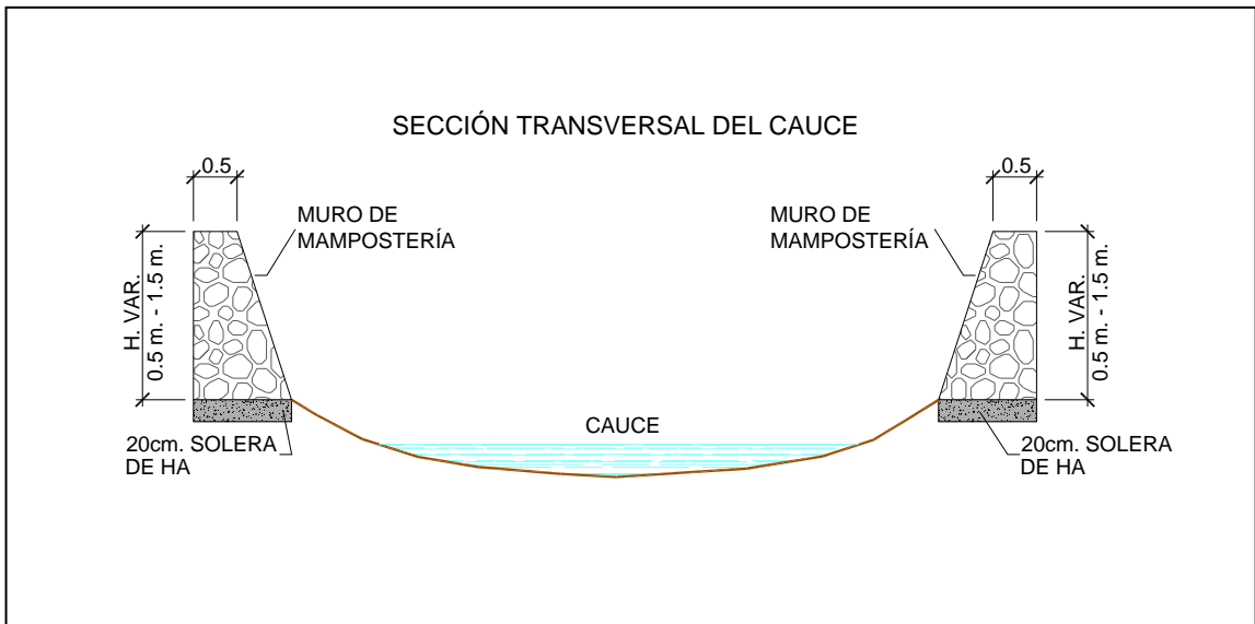
Sección tipo del encauzamiento en el tramo previo al cruce con la N-332
