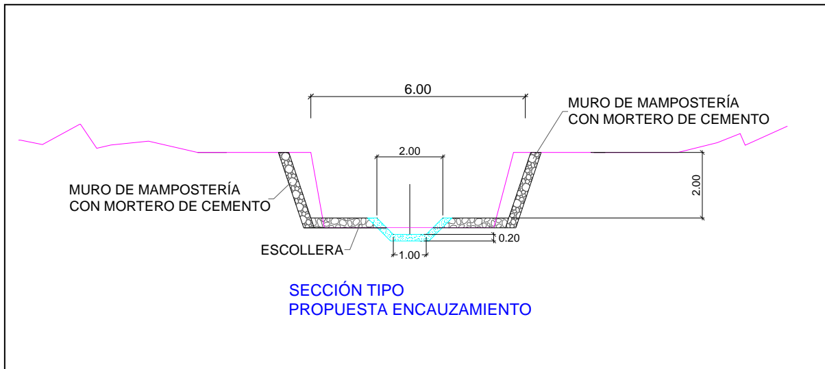
Sección tipo ALF-ENC01
