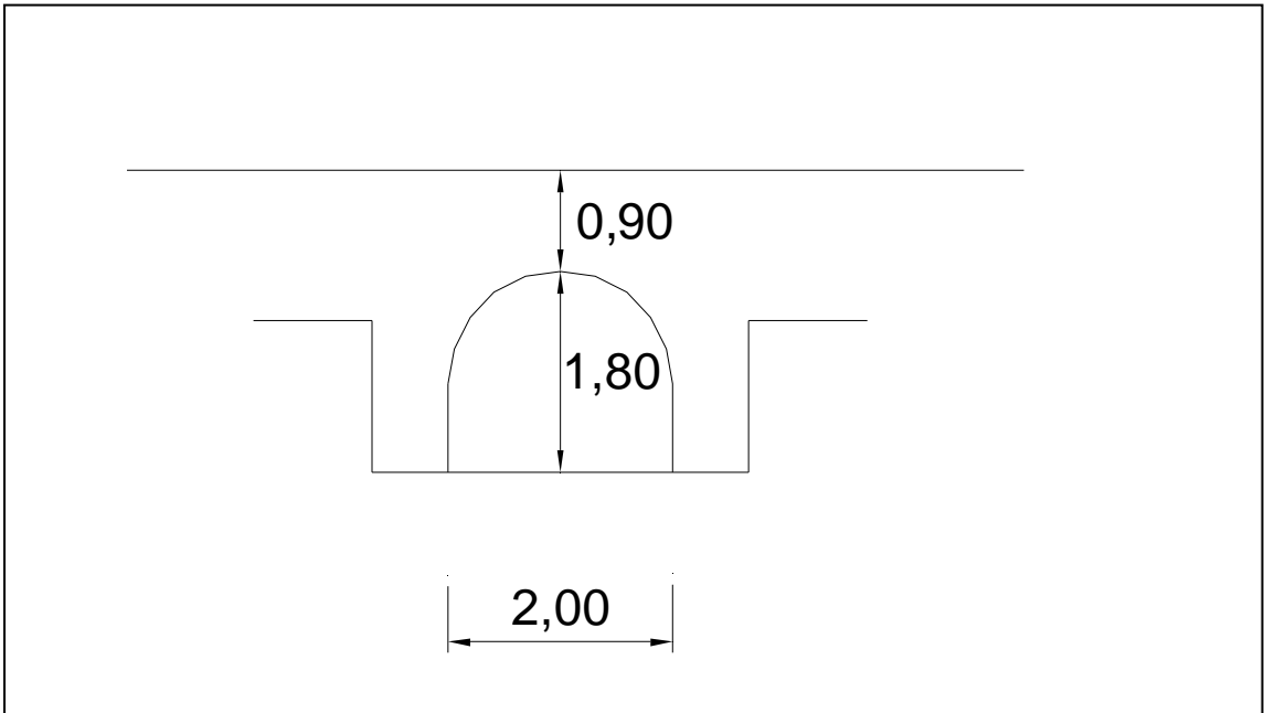
Croquis situación actual de la obra de paso ALF-109
