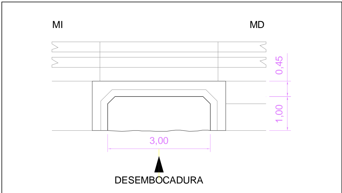
Croquis situación actual de la obra de paso ALF-107
