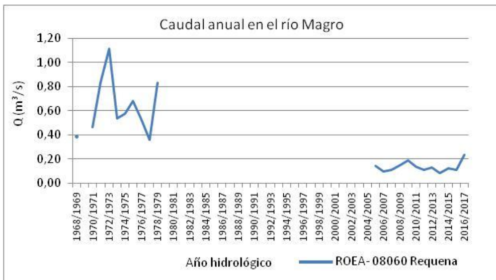
Figura 7 Serie histórica de caudales ( m^3/s ) anuales en la estación de aforos 08060- Requena, en el río Magro
