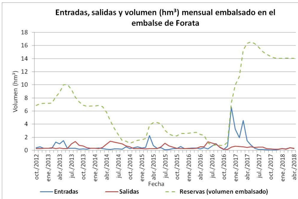
Figura 5 Embalse de Forata: entradas, salidas y volumen mensual embalsado de los 5 últimos años.
