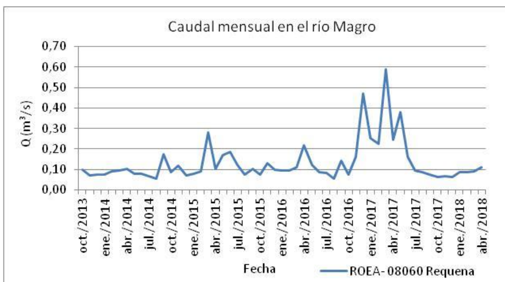
Figura 8 Serie de caudales ( m^3/s ) mensuales de los 5 últimos años en la estación de aforos 08060- Requena, en el río Magro
